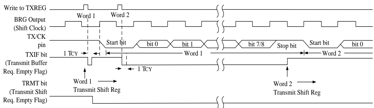
Рис. 3.8. Временная диаграмма асинхронной передачи по EUSART байт «один за одним»
