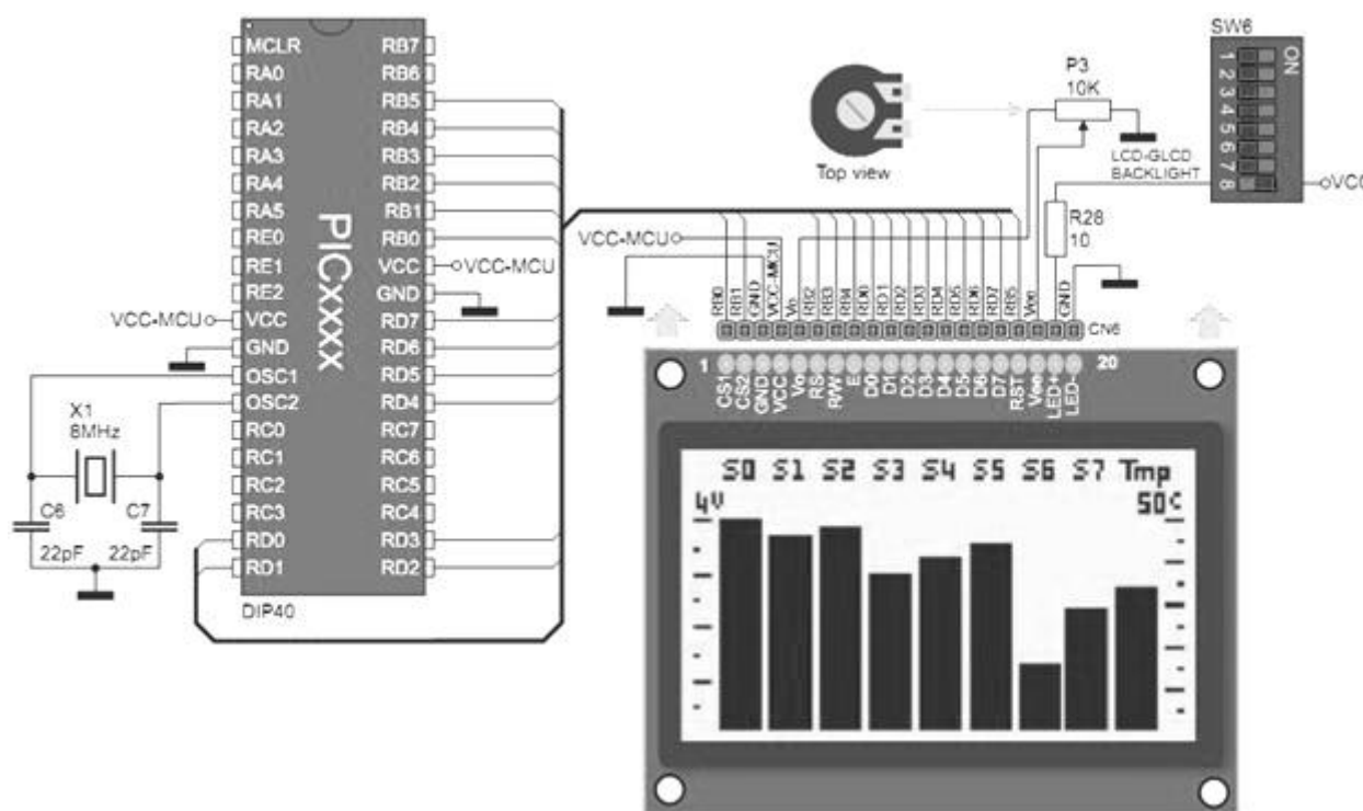
Рис. 2.6 Принципиальная электрическая схема подключение графического ЖК-дисплея
