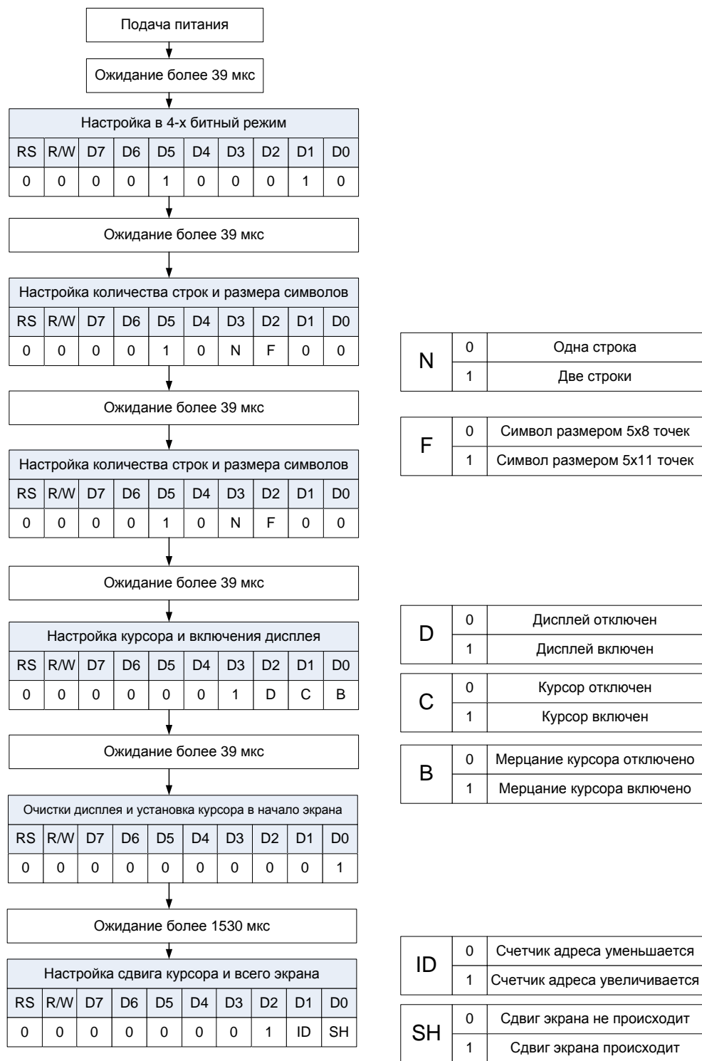
Рис. 2.1. Инициализация контроллера KS0066 в 4-х битный режим работы
