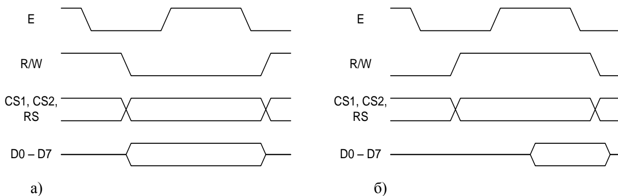
Рис. 2.4. Общий вид временных диаграмм сигналов чтения и записи контроллера KS0107 или аналогичного: а) запись данных, б) чтение данных
