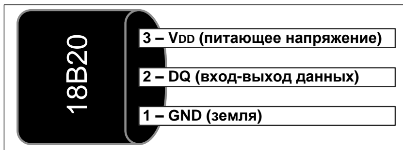
Рис.4.2. Цифровой термометр DS18B20
