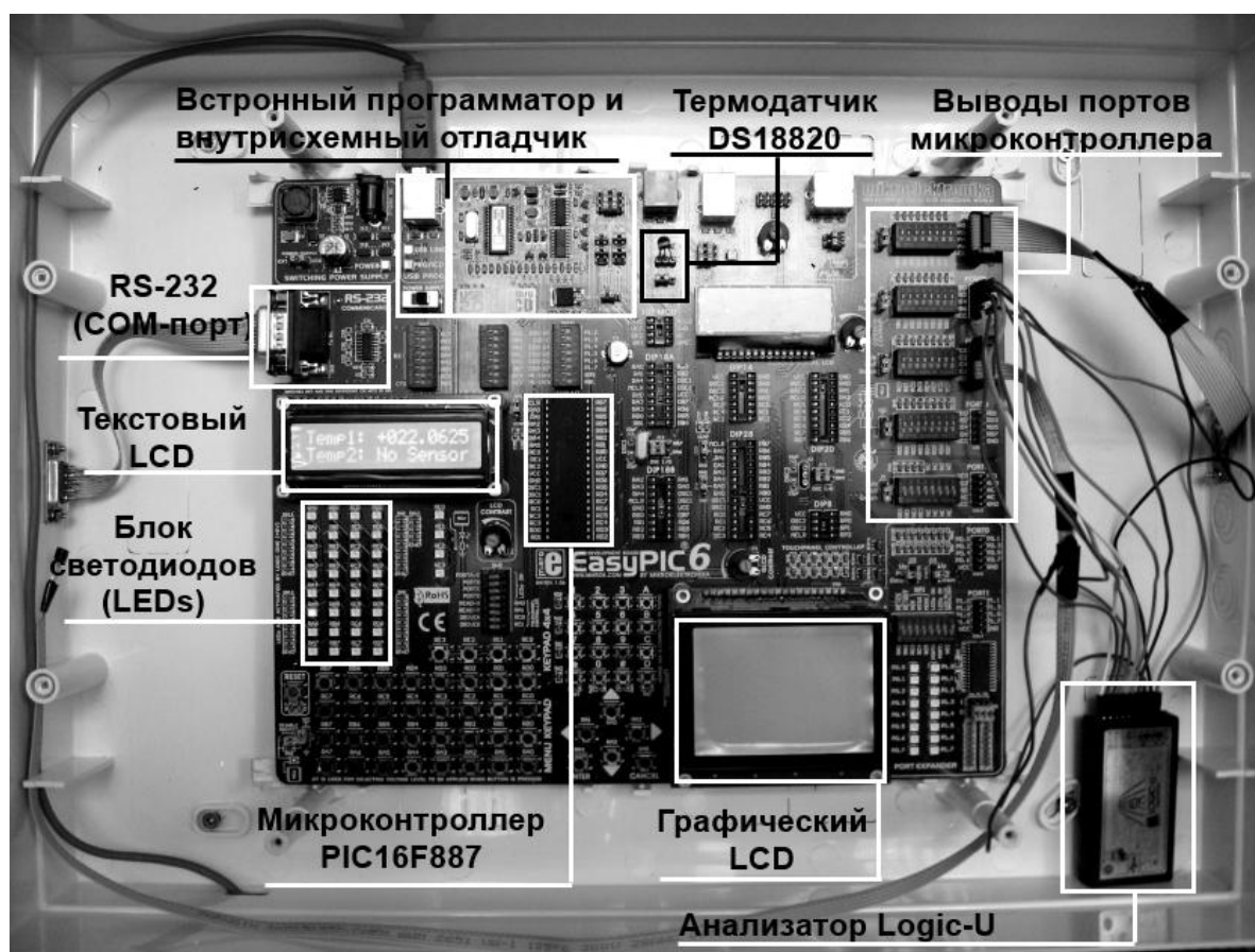
Рис. 1. Внешний вид лабораторного макета
