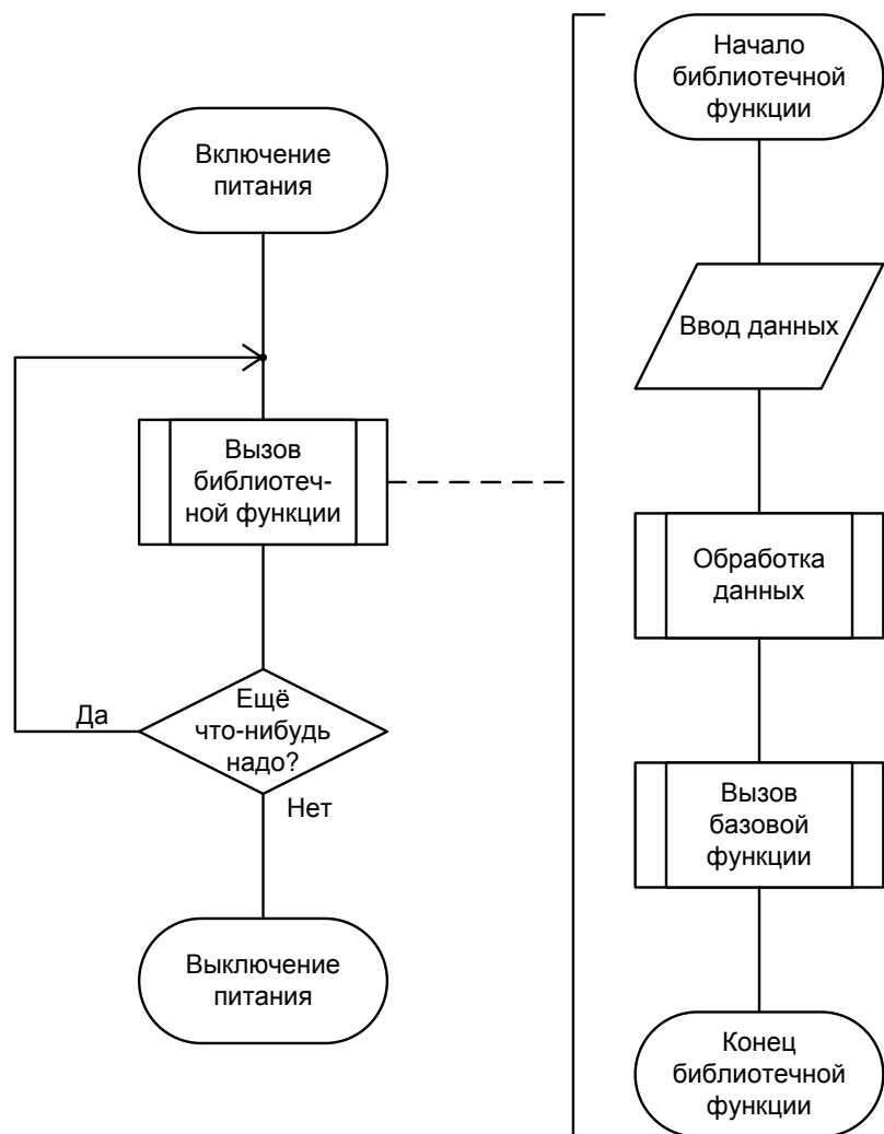
Рис.2.3. Общий вид алгоритма управления графическим ЖК-дисплеем WDG0151
