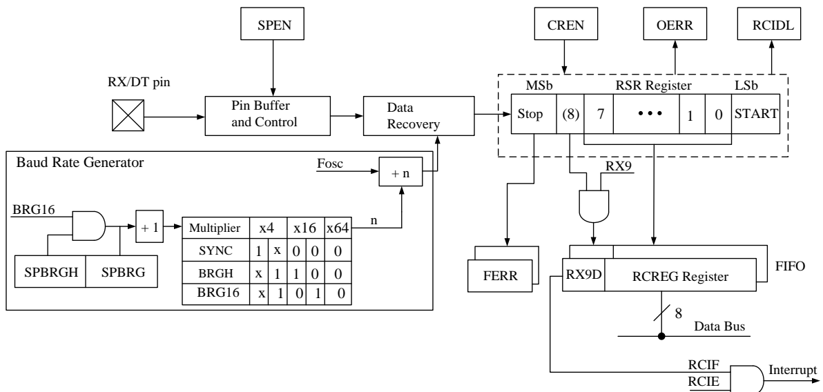
Рис. 3.6. Структурная схема приемника EUSART
