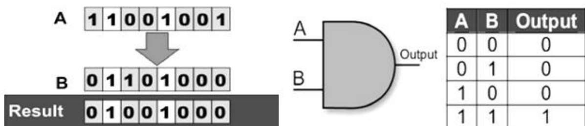
Рис. 1.14 Логический элемент И.
