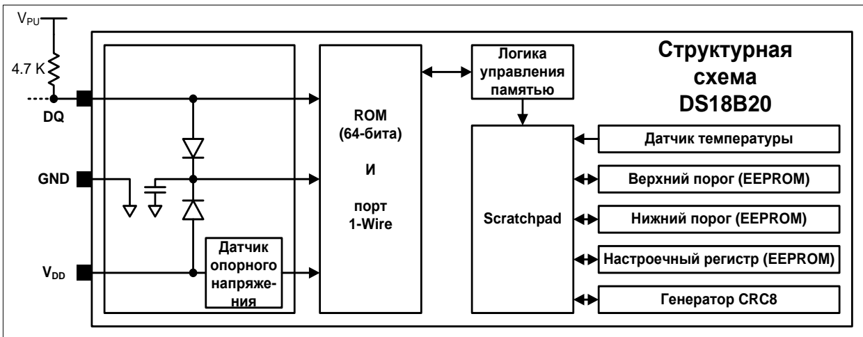
Рис.4.3. Структурная схема цифрового термометра DS18B20
