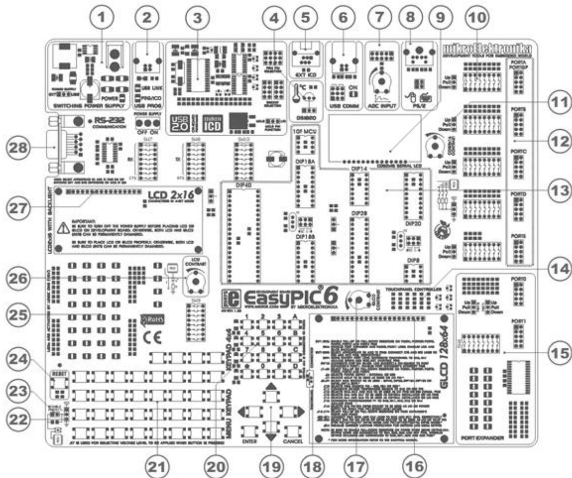
Рис. 1.55 Расположение периферии на платформе EasyPIC6
