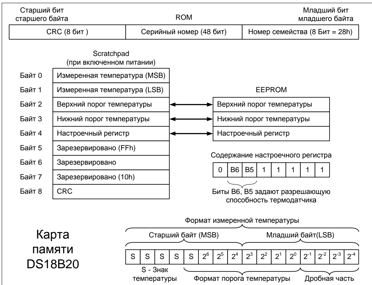
Рис.4.4. Карта памяти цифрового термометра DS18B20
