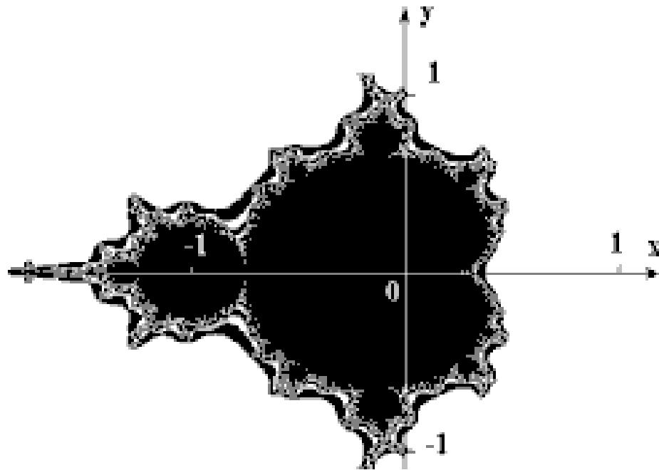
Рис. 4.3. Множество Мандельброта
