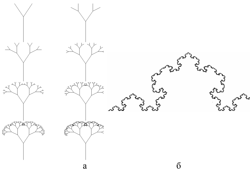
Рис. 4.5. Методы построения фракталов: а – пример построения дерева с помощью L-системы; б – изображение кривой Коха, полученное с использованием IFS
