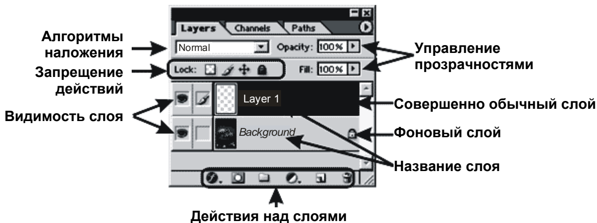
Рис. 3.2. Параметры слоев
