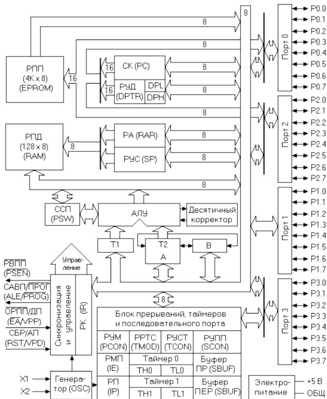
Рис. 16. Структурная схема микроконтроллера 1816BE51
