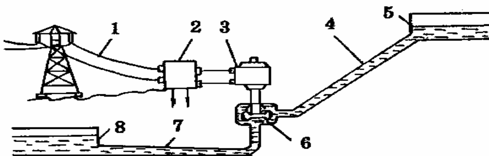
Рис.3.6 Схема гидроаккумулирующей электростанции.
