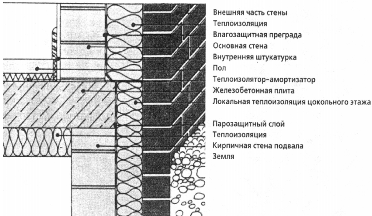
Рис.8.5 Сокращение теплопотерь в цокольном этаже при неотапливаемом подвале
