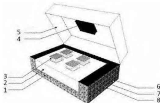
Рисунок 1 – Макет устройства исследовательской установки CN 106597569 А
