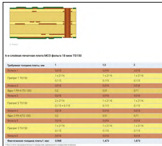
Рисунок 2 – Типовая структура шестислойной платы
