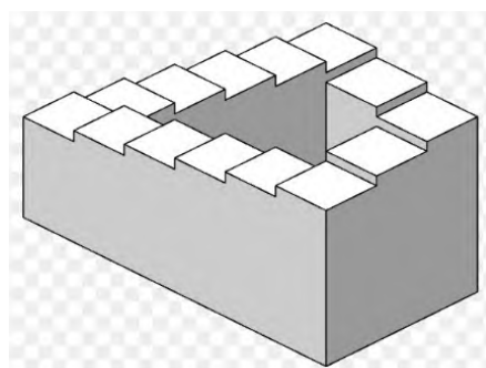
Рисунок 2 – Лестница Пенроуза
