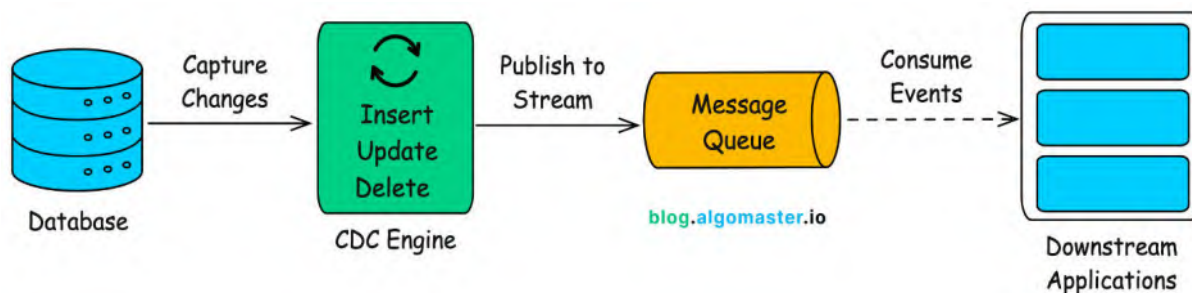
Рисунок 1 – Паттерн CDC
