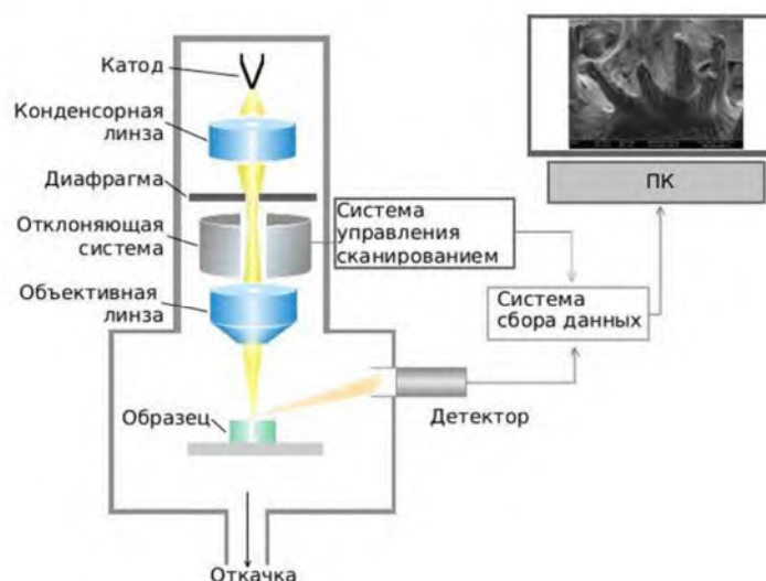
Рисунок 1 – Принципиальная схема СЭМ
