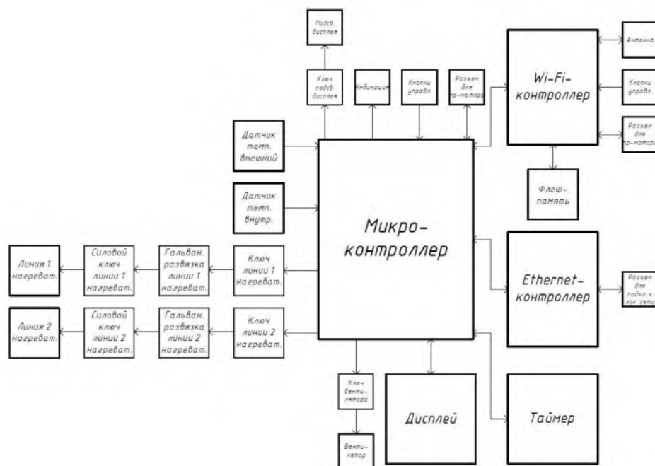
Рисунок 1 – Структурная схема устройства
