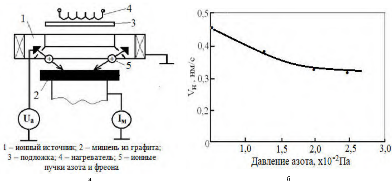
Рисунок 1 – Схема реактивного ионно-лучевого формирования фторуглеродных покрытий (а) и зависимость скорости нанесения от парциального давления азота (б)
