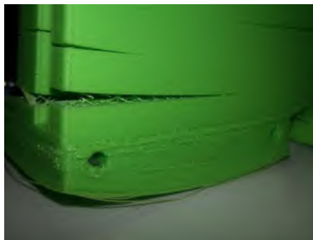
Рисунок 2 – Расслоение вдоль слоев
