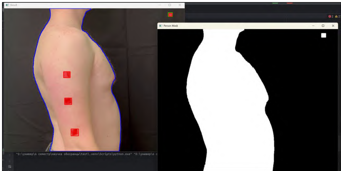
Рисунок 1 – Выделение маски
