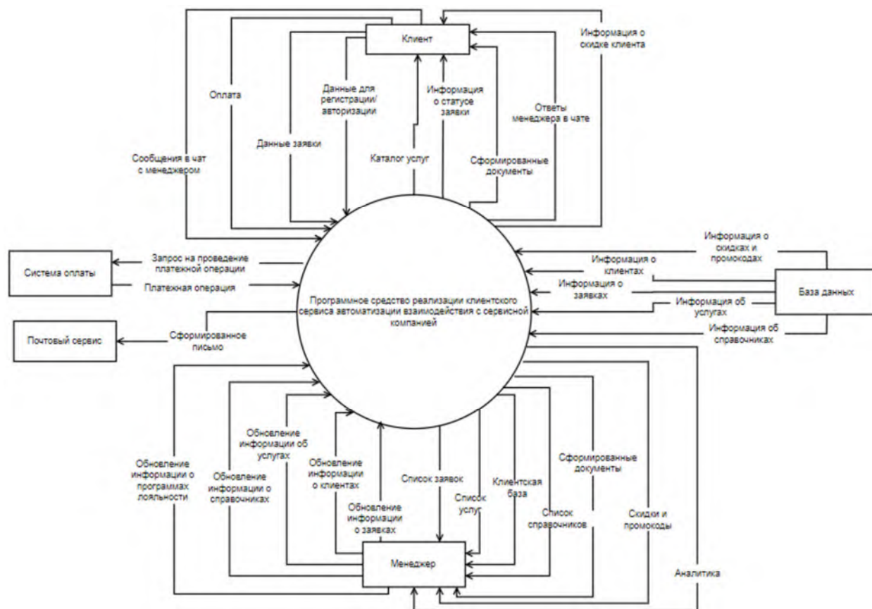
Рисунок 2 – Контекстная диаграмма
