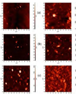
Рисунок 6 - АСМ-изображения PDA/AU [8]
