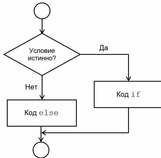
Рисунок 2.3 – Алогритм работы оператора условия
