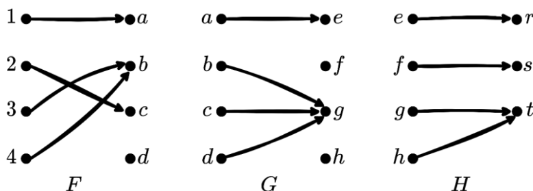
Рисунок 3.4 – Графы функций F, G и H для задачи 13 раздела 3
