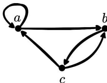
Рисунок Б.9 – Ответ к задаче 14 раздела 2
