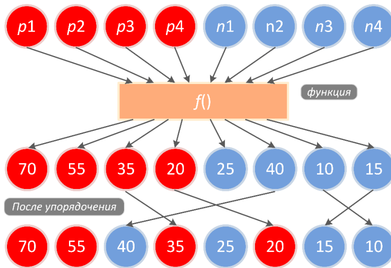
Рисунок 2.6 – Введение отношения порядка на множестве
