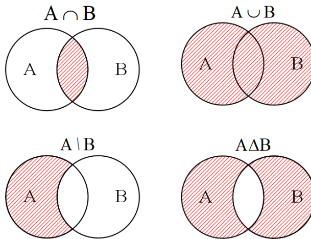
Рисунок 1.1 – Примеры использования кругов Эйлера
