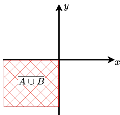
Рисунок А.1 – Ответы к задаче 13 раздела 1: a – A \cap B ; б – A \cup B ; в – A \setminus B ; г – \bar{A} ; д – \overline{A \cap B} ; е – \overline{A \cup B}
