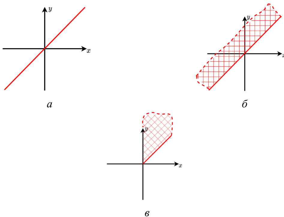
Рисунок Б.2 – Ответы к задаче 3 раздела 2
