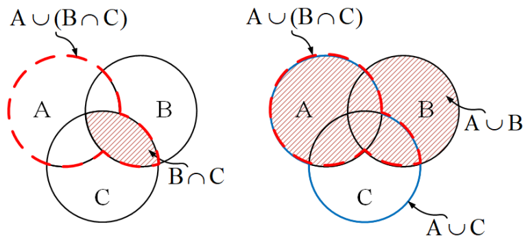
Рисунок 1.2 – Круги Эйлера для примера 1.8
