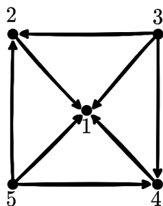
Рисунок 2.13 – Граф для задачи 19 раздела 2
