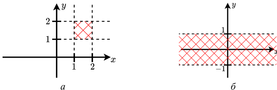
Рисунок Б.1 – Ответы к задаче 2 раздела 2
