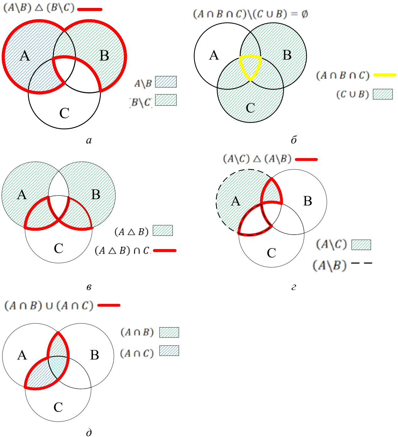
Рисунок А.2 – Ответы к задаче 23 раздела 1
