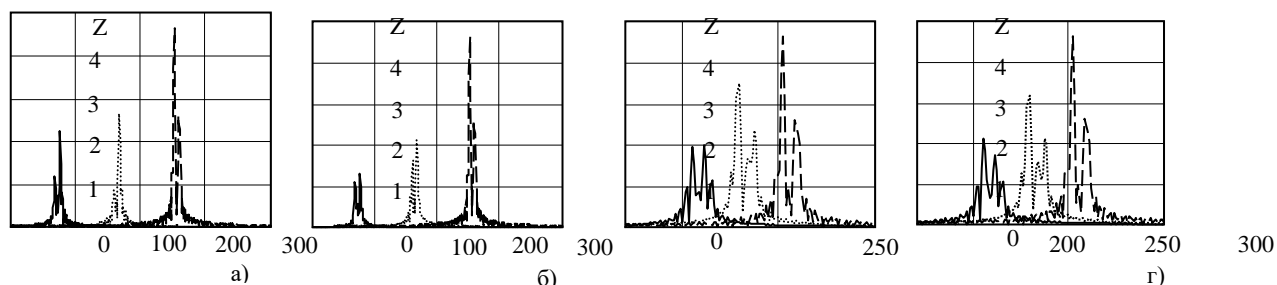
Рисунок 5 – Пример отраженного цели тип-1 сигнала на выходе ВПО при времени наблюдения T_{\text{КН}}=1 с (а,б) и при T_{\text{КН}}=256 мс (в,г) в случаях без учета атмосферы (а,в) и турбулентности ясной погоды (б,г). (длинный штрих – k=0 ; круглые точки k=500 (а,б), 128 (в,г); сплошная линия k=999 (а,б), 255 (в,г))
