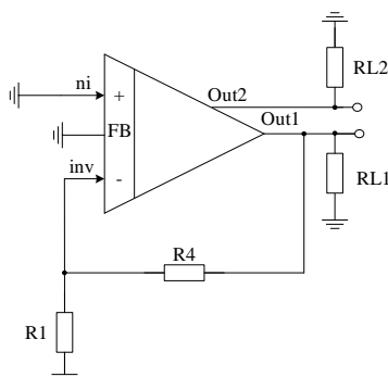
Рисунок 3 – Схема включения OАmp2 при определении напряжения смещения нуля. V_{OFF} = -V_{OUT1}/(R4/R1+1) , R1 = 83 Ом, R4=128 кОм, RL1 и RL2 не подключены
