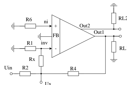
Рисунок 4 – Схема включения OАmp2 при определении коэффициента усиления напряжения. K_V = (R_x/R1) \cdot (V_{OUT1}/V_x) , R1=R6= 475 Ом, R2=R4=10 кОм, R_x=118 кОм, RL1 и RL2 не подключены, V_{IN} = 1 В (p-p), f_{IN} = 100 Гц
