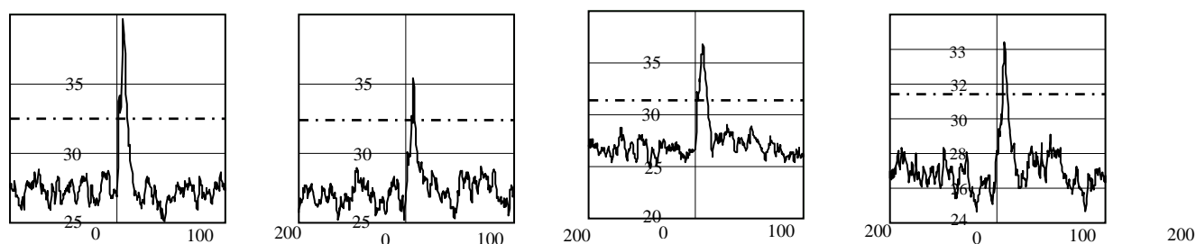
Рисунок 4 - Результат комбинированного накопления при периоде рысканий 2, 1, 0,5 и 0,25 с
