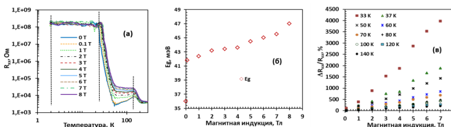
Рисунок 1 – (а) Температурные зависимости продольного сопротивления R xx в геометрии Ван дер Пау при различных магнитных полях от 0 Тл до 8 Тл; (б) Зависимость ширины запрещенной зоны в диапазоне температур 25-50 К от магнитной индукции; (в) зависимость относительного магнитосопротивления от магнитной индукции при температурах от 33 К до 140 К
