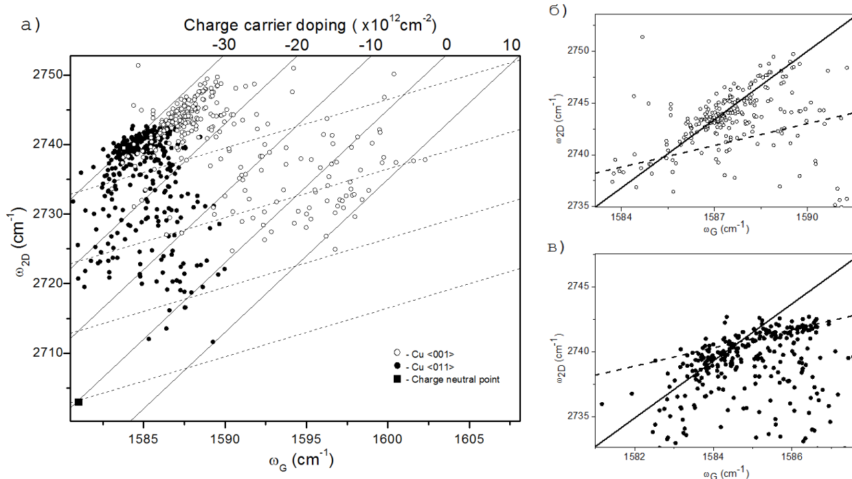
Рисунок 3 – Экспериментальные зависимости положения линии 2D от положения линии G для всех исследуемых образцов (а); экспериментальные зависимости положения линии 2D от положения линии G для образцов графена, выращенных на медном катализаторе с ориентацией \langle 001 \rangle (б) и \langle 011 \rangle (в); Линии постоянного напряжения и постоянной концентрации носителей заряда проведены согласно работе [2] и [3] соответственно
