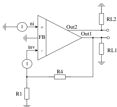
Рисунок 2 – Схема включения OАmp2 при измерении тока потребления и входных токов. I -АКИП-2101/2, R1 = 1,18 кОм, R4=10 кОм, RL1 и RL2 не подключены
