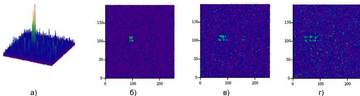
Рисунок 1 - Трехмерное (а) и яркостное (б-г) РЛИ цели в координатах дальность-доплеровский сдвиг частоты при точном (а, б) согласовании параметров системы обработки и рассогласовании по ускорению 20 м/с 2 (в) и 40 м/с 2 (г)
