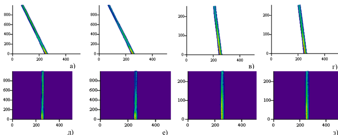
Рисунок 7 – Яркостное РЛИ на выходе ВПО в виде сигналов до (а-г) и после (д-з) компенсации миграции дальности при времени наблюдения T_{\text{КН}}=1 с (а, б, д, е) и при T_{\text{КН}}=256 мс (в,г, ж, з) в случаях без учета атмосферы (а, в, д, е) и турбулентности ясной погоды (б, г, е, з)
