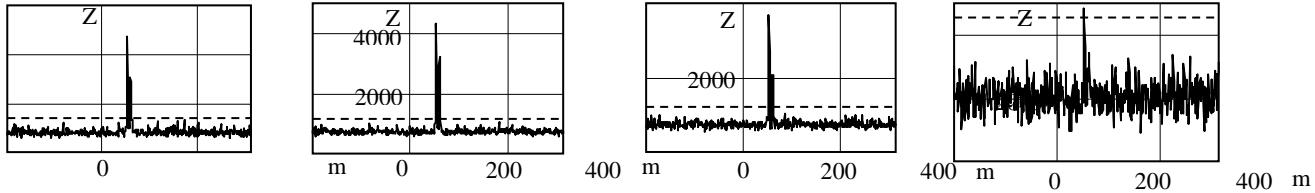
Рисунок 10 - Результат комбинированного накопления при изменении числа подпачек, на которые разбивается пачка Q_1=2 (а), Q_1=10 (б), Q_1=4 (в) и некогерентного накопления (г).
