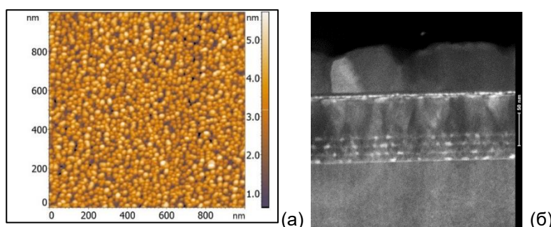
Рис.1. (а) АСМ изображение массива нанокристаллов GaSb на Si(111). Концентрация НК 2.2 \times 10^{11} \text{ см}^{-2} , средний латеральный размер 15 нм, высота 1.7 нм. (б) Снимок ПЭМ гетероструктуры Si/НК GaSb/Si.
