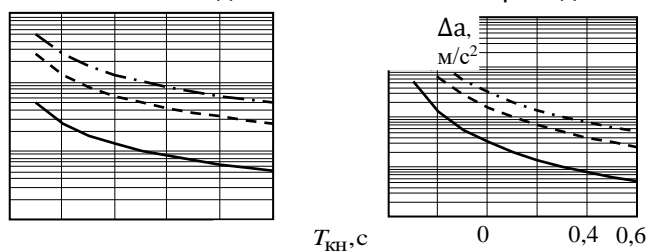
а) б) Рисунок 1- Зависимость разрешающей способности по скорости (а) и ускорению (б) для различных значений длины волны (сплошная кривая - \lambda = 1 см, пунктирная - \lambda = 5 см, штрихпунктирная - \lambda = 10 см)
