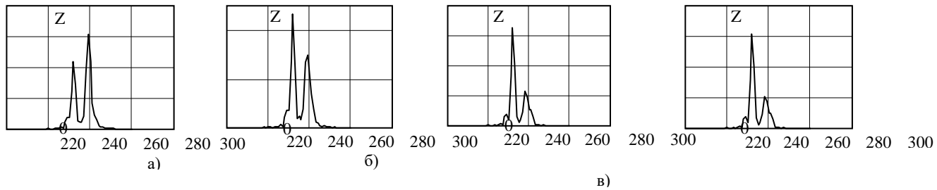
Рисунок 9 - Результат некогерентного накопления при времени накопления T_{\text{КН}} = 1 с (а,б) и при T_{\text{КН}} = 256 мс (в,г) в случаях без учета атмосферы (а,в) и турбулентности ясной погоды (б,г)
