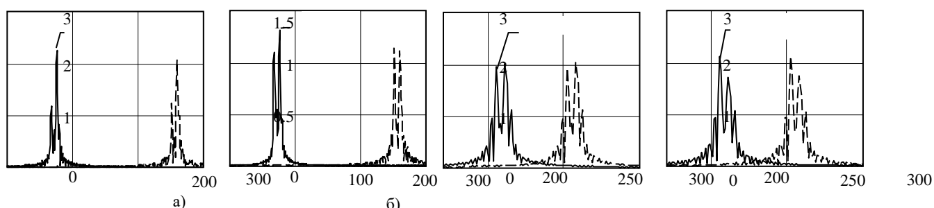
Рисунок 6 – Сигнал на выходе ВПО до (сплошная линия) и после (длинный штрих) компенсации миграции дальности при времени наблюдения T_{\text{КН}}=1 с (а,б) и при T_{\text{КН}}=256 мс (в,г) в случаях без учета атмосферы (а,в) и турбулентности ясной погоды (б,г)
