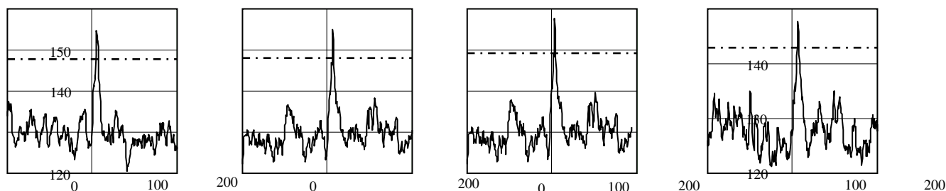
Рисунок 3 - Результат некогерентного накопления при периоде рысканий 2, 1, 0,5 и 0,25 с
