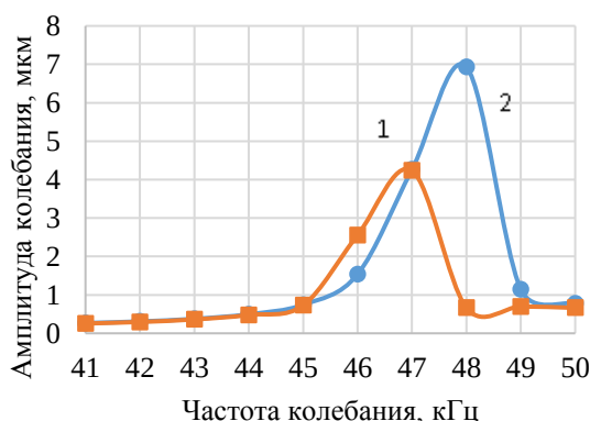
1 – соединение клеем ; 2 – с паяным соединением Рисунок 6 – АЧХ инструмента микросварки в пакете ANSYS:
