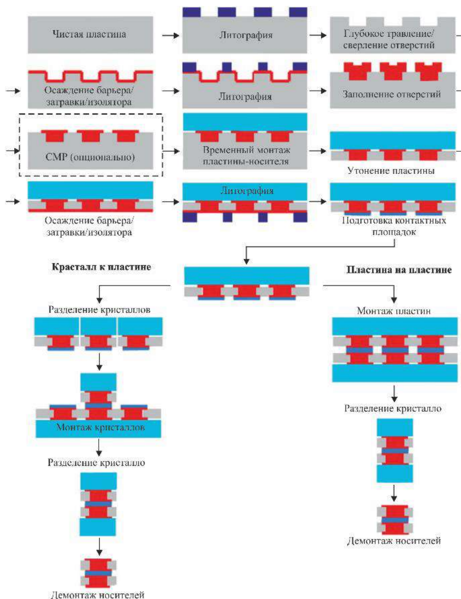
Рисунок 2. – Типовой технологический процесс производства 3D ИС [2]
