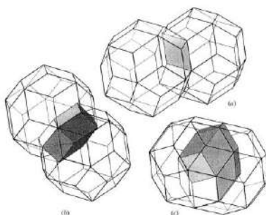
Рисунок 2 – Три способа объединения тетраэдров в трехмерную квазикристаллическую структуру
