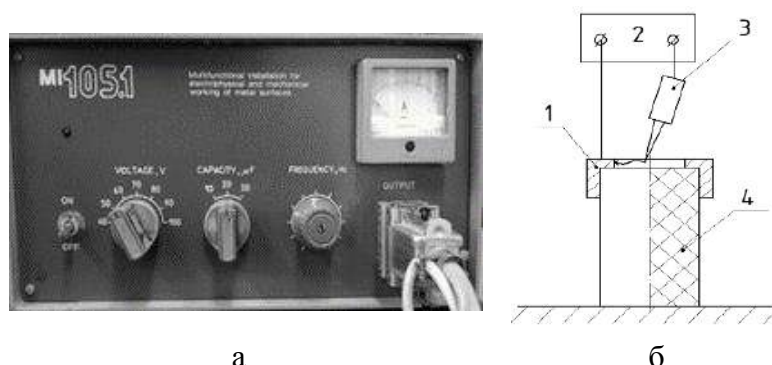
1 – кольцо, 2 – генератор импульсов, 3 – медный электрод, 4 – ферритовый стержень Рисунок 2 – Генератор импульсов зарядов MI105.1(а), схема процесса электроискровой обработки феррита (б):
