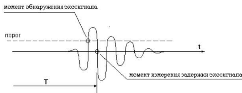
Рисунок 1 – Измерение задержки ультразвукового сигнала методом перехода через ноль [2]
