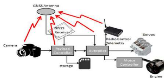
Рисунок 1 – Типичные электронные системы БПЛА
