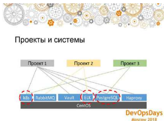
Рис.1 - Взаимодействие программы и сервисов в проекте IaC
