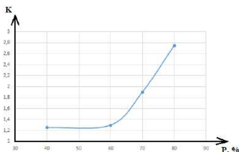
Рисунок 6 – Зависимость коэффициента K = I_{\text{ток}} / I_{\text{опт.}} от мощности
