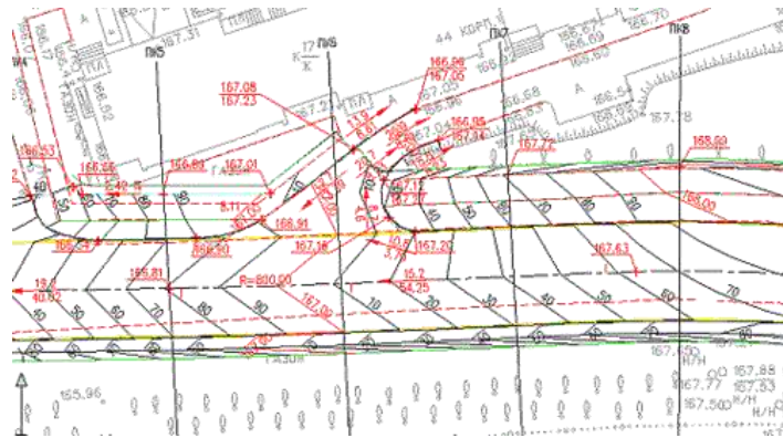
Рисунок 2 – Вертикальная планировка трассы
