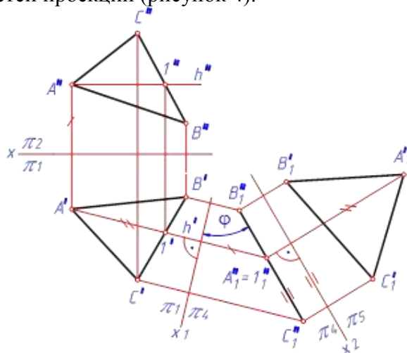
Рисунок 1 - Способ замены плоскостей проекций
