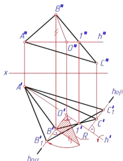
Рисунок 2 - Способ вращения вокруг линии уровня
