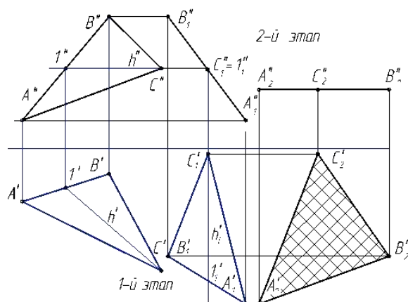
Рисунок 1 - Способ замены плоскостей проекций
