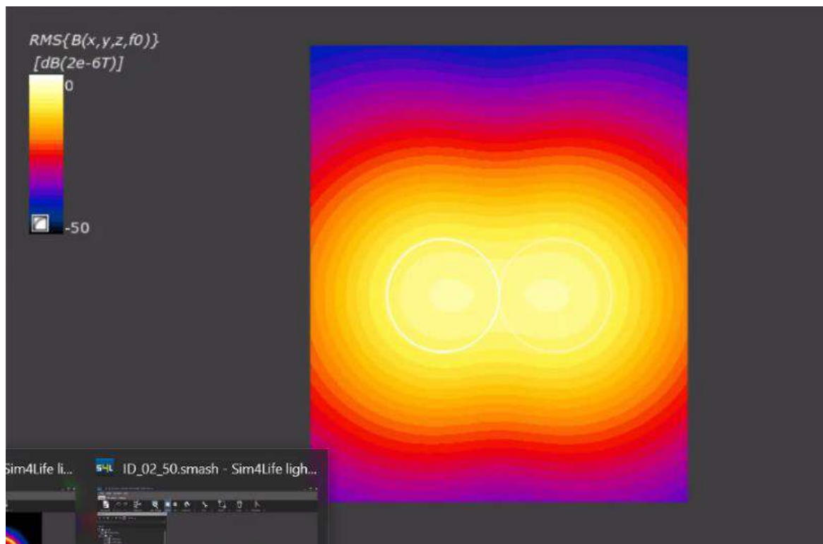
Рисунок 2 – Распределение магнитной индукции
