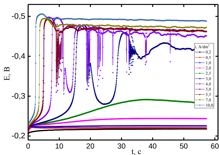
Рисунок 1 – Зависимость «потенциал–время»
