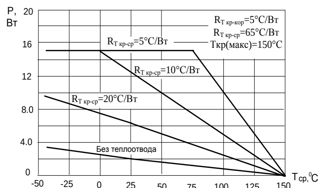
Рисунок 3. – Зависимость допустимой мощности рассеивания полупроводниковых приборов и ИМС силовой электроники от температуры среды для разных условий теплоотвода (корпус ТО – 220)
