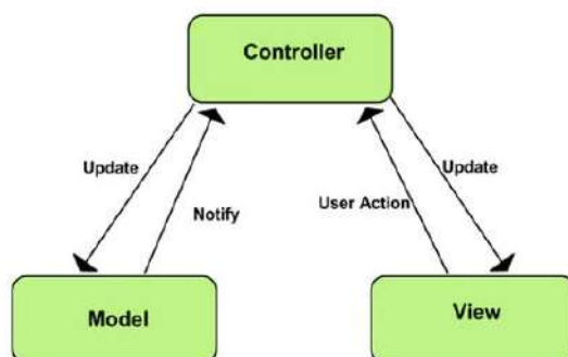
Рисунок 1 – Схема взаимодействия компонентов MVC
