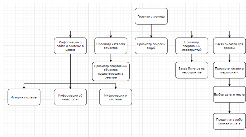
Рисунок 1 – структурная схема разрабатываемого web-ресурса
