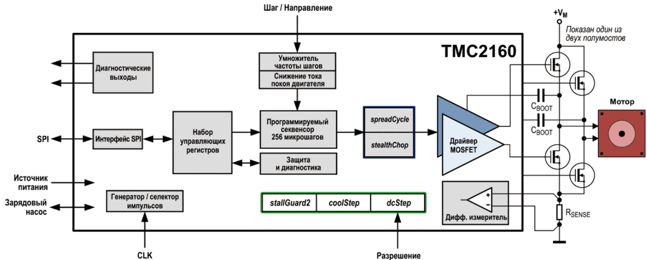
Рисунок 2 – Архитектура драйвера шагового двигателя
