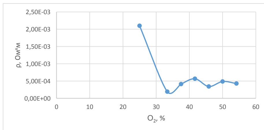
Рисунок 2 – Зависимость удельного сопротивления тонких пленок второго эксперимента от концентрации кислорода в \text{Ar}/\text{O}_2 смеси газов
