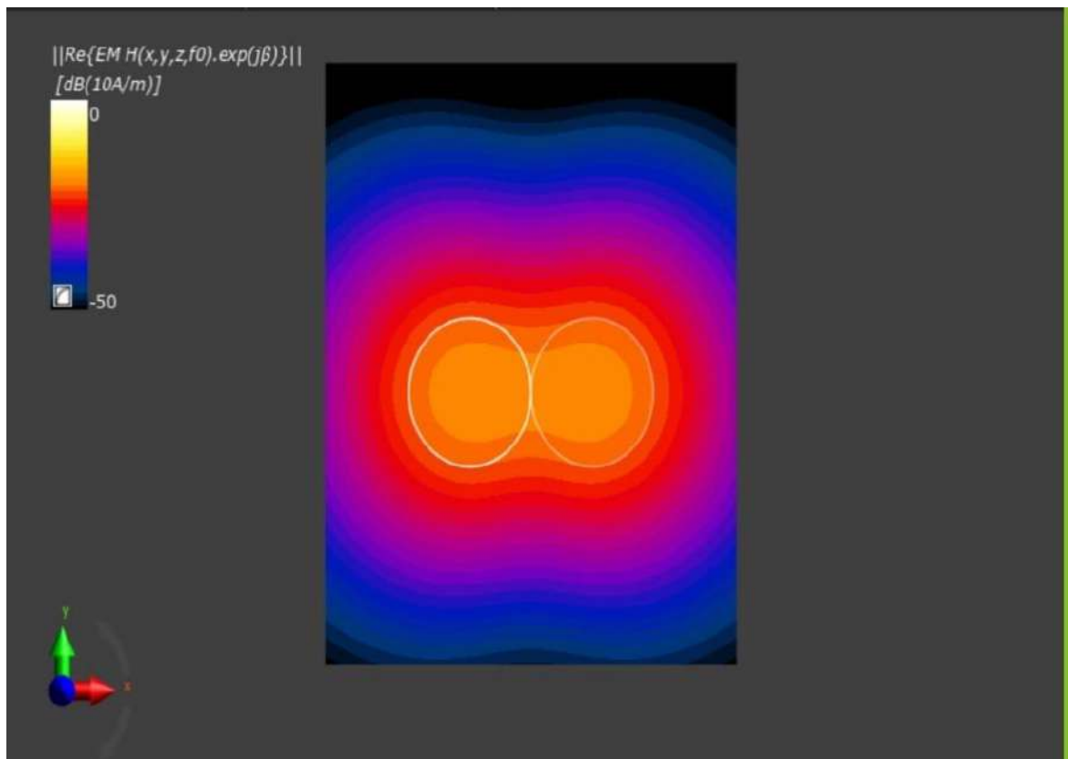
Рисунок 1 – Распределение магнитной составляющей электромагнитного поля
