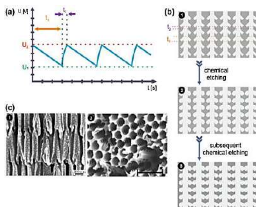
Рисунок 3 – Схематическая иллюстрация процесса синтеза пористого АОА с периодически разветвленными нанопорами. Типичный сигнал напряжения, подаваемый при периодическом анодировании алюминия (а). Схематическое представление структуры АОА, выращенной после (1) нескольких циклов периодического анодирования и (2, 3) последующего химического травления (b). СЭМ-микрофотография, показывающая поперечные сечения подготовленных слоев АОА методом (1) периодического анодирования и (3) после последующего химического травления (с)
