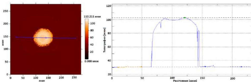
Рисунок 7 – Припойный бамп SAC, измеренный прибором MicroProf с программным обеспечением Mark III
