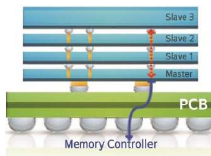
Рисунок 1 – Реализация 3D-модуля по технологии TSV
