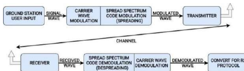
Рисунок 1 – Модуляция с расширенным спектром [1]
