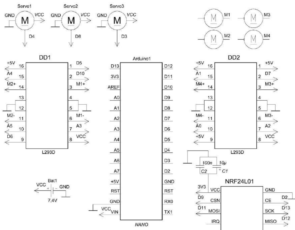
Рисунок 2 – Схема модуля-приемника
