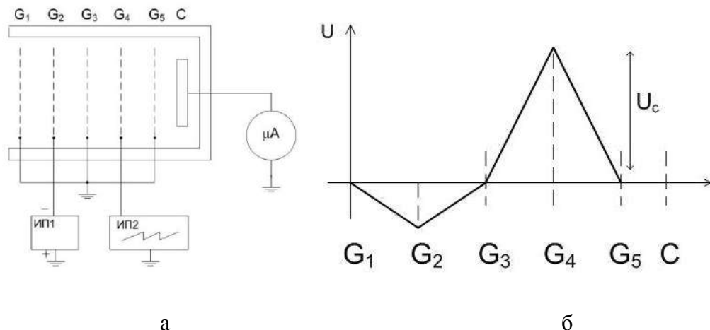
Рисунок 2 – Упрощенная схема шестиелектродного электростатического зонда ENPR.412-01 (а) и распределение потенциалов на сетках зонда (б)
