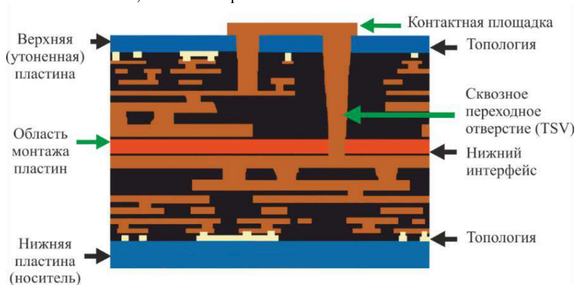
Рисунок 1. - Типовая конструкция микросборки, выполненной с использованием технологии TSV
