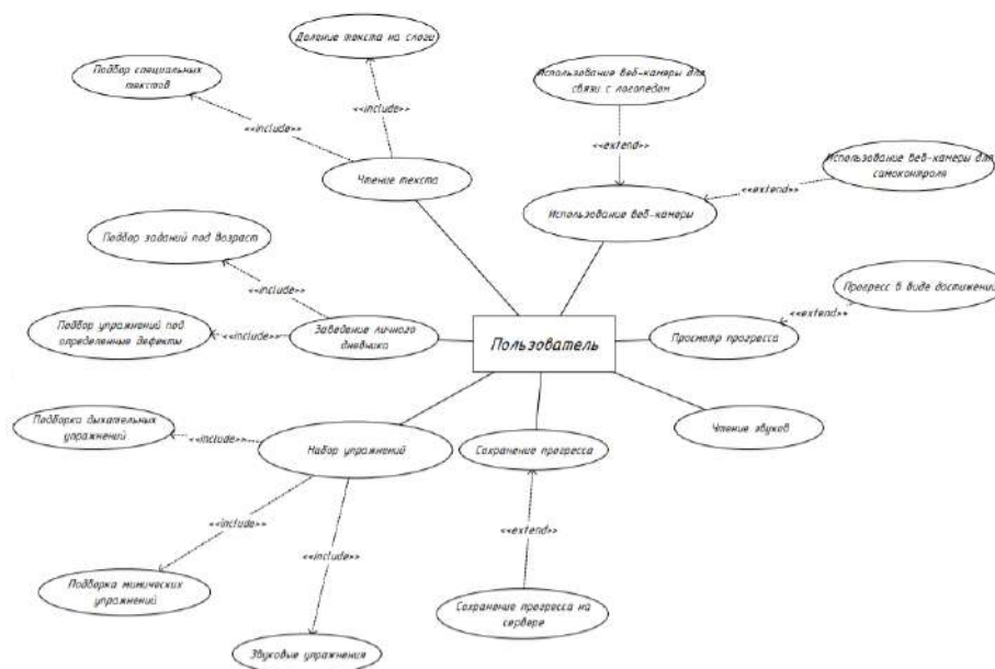
Рисунок 1 – Диаграмма вариантов использования веб-ресурса.
