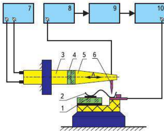
1 – контактная площадка; 2 – проволочный вывод; 3 – система крепления; 4 – пьезоэлектрический преобразователь; 5 – волновод; 6 – сварочный капилляр; 7 – генератор УЗ колебаний; 8 – блок питания; 9 – блок управления; 10 – устройство токовой активации
