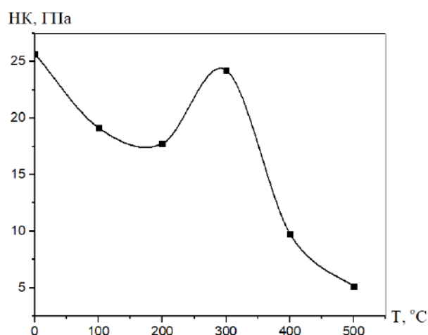
Рисунок 2 – Зависимость микротвердости пленок \text{Ti}_x\text{Zr}_{1-x}\text{N}_y от температуры отжига
