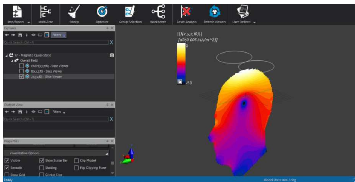
Рисунок 3 – Распределение плотности тока
