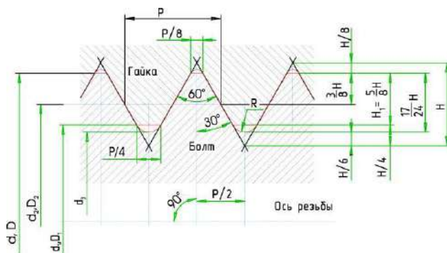
Рисунок 1 – ГОСТ 24705.81 Основные размеры
