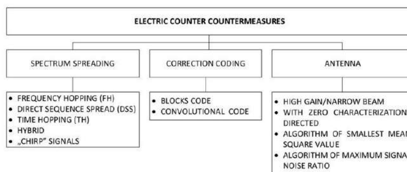
Рисунок 2 – Классификация механизмов, иммунизирующих радиостанции от преднамеренных помех [2]
