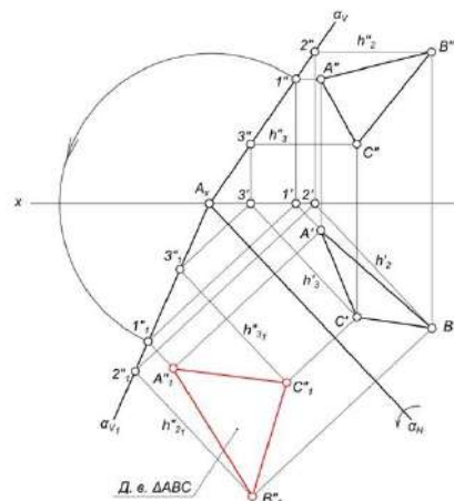
Рисунок 2 - Способ вращения вокруг линии уровня
