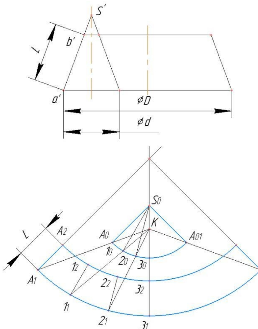
Рисунок 2 – Развёртка конуса вращения с недоступной вершиной
