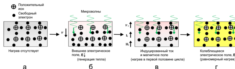
Рисунок 1 – Механизм нагрева при потерях на проводимость
