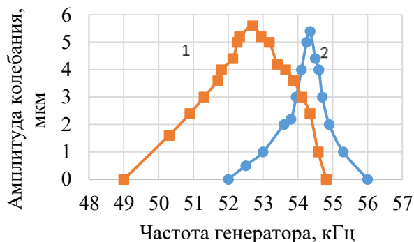
1 – с клевым соединением; 2 – с паяным соединением Рисунок 4 – АЧХ магнитострикционного преобразователя.
