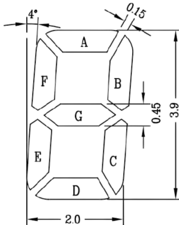
Рисунок 2 – Схема последовательности сегментов разряда на дисплее
