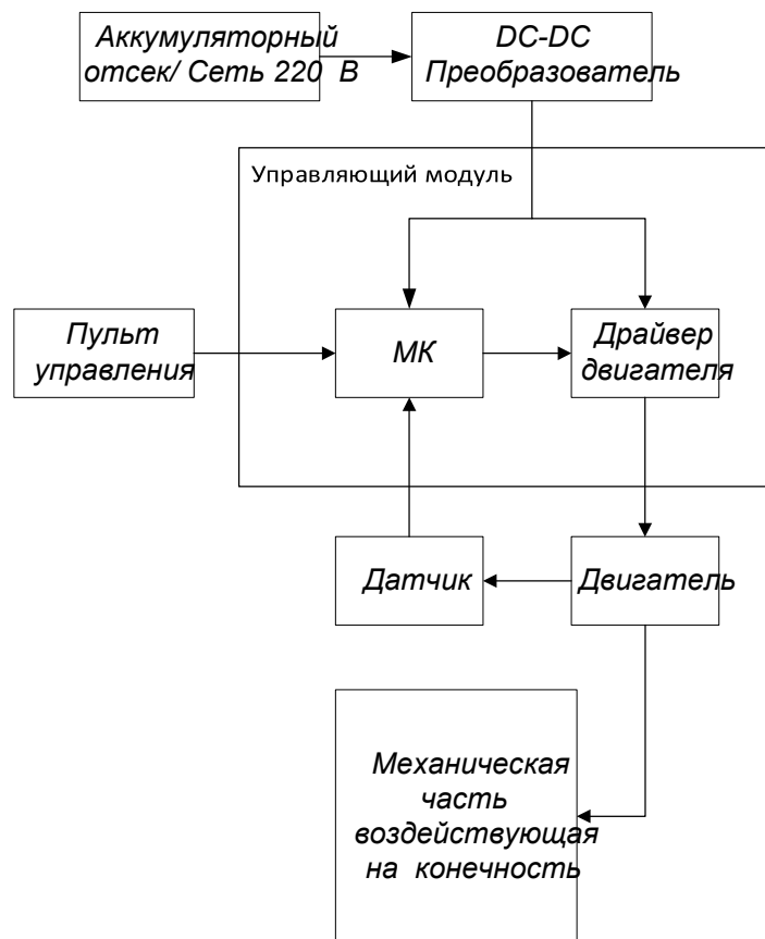
Рисунок 1 – Общая схема мобильной роботоплатформы
