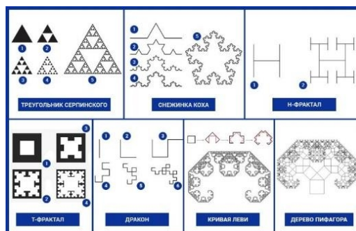
Рисунок 2 – Геометрические фракталы
