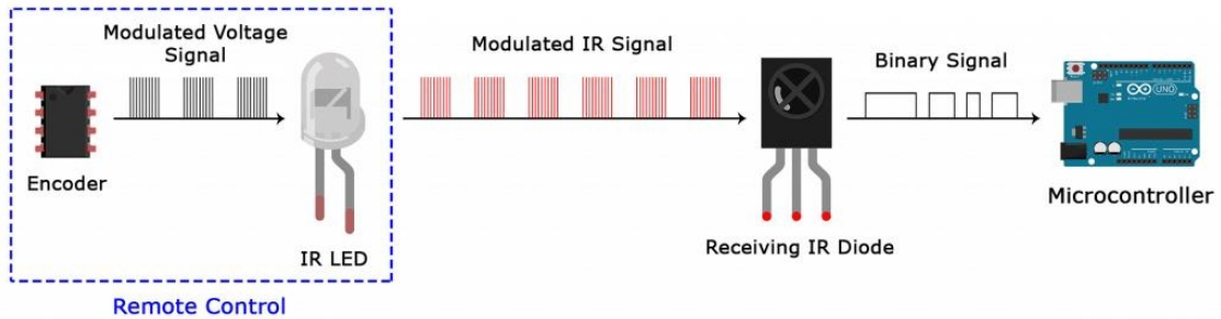
Рисунок 1 – Схема передачи сигнала от пульта к микроконтроллеру
