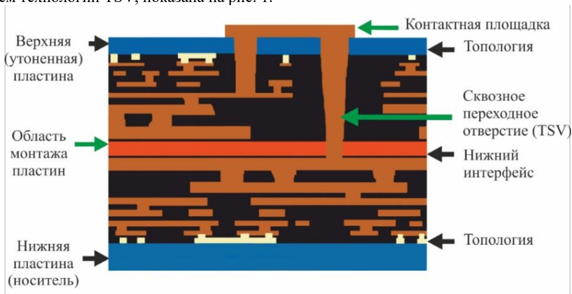
Рисунок 1. - Типовая конструкция микросборки, выполненной с использованием технологии TSV
