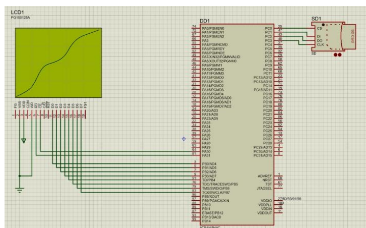
Рисунок 1 – Схема соединения микроконтроллера ATMEGA328P с дисплеем PG160128A
