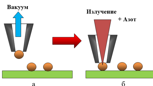
Рисунок 2 – Припойный шарик перед присоединением под торцом сварочного инструмента (а); припойный шарик в позиции присоединения (б)
