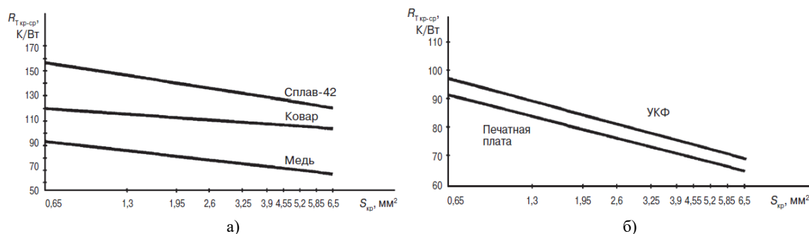
Рисунок 5. – Зависимость теплового сопротивления от площади кристалла для корпуса DIP 16: а) от материала кристаллодержателя; б) для двух способов монтажа (пайки на печатную плату или устройство контактирования УКФ)
