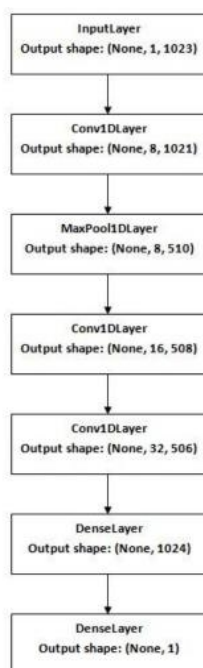
Рисунок 2 - Архитектура нейронной сети
