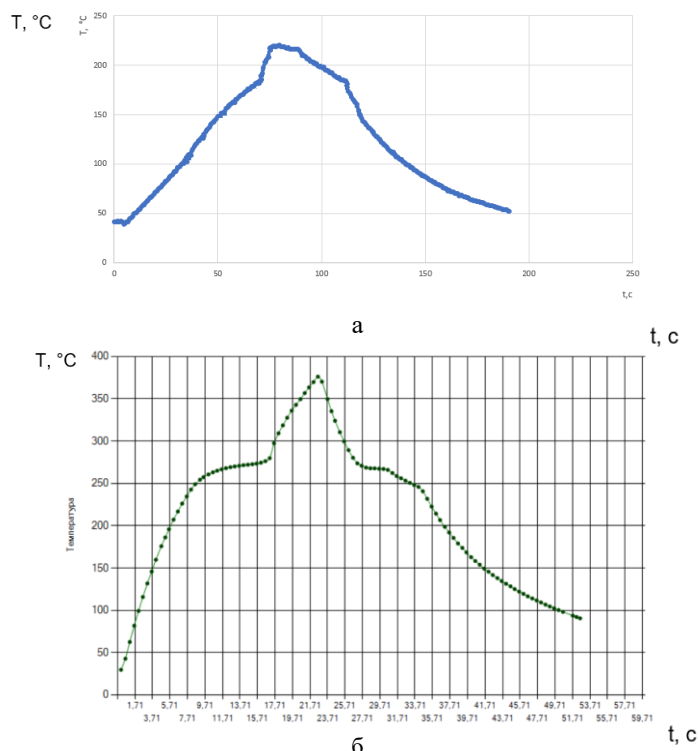
Рисунок 3 – Термограммы процесса ВЧ пайки, созданные с помощью: а – пакета Excel б – созданная с помощью ПО системы
