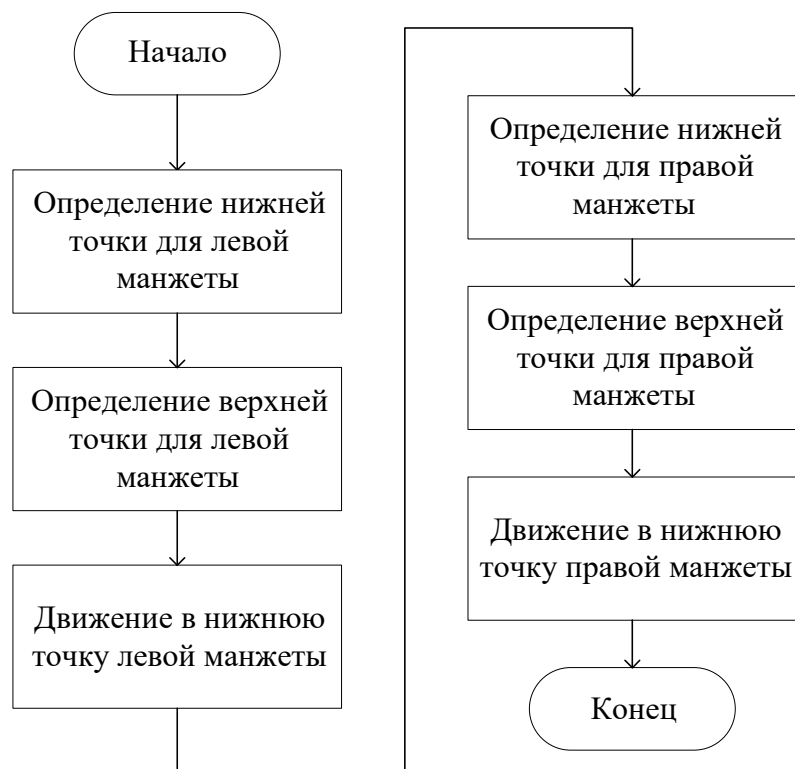
Рисунок 2 – Алгоритм калибровки
