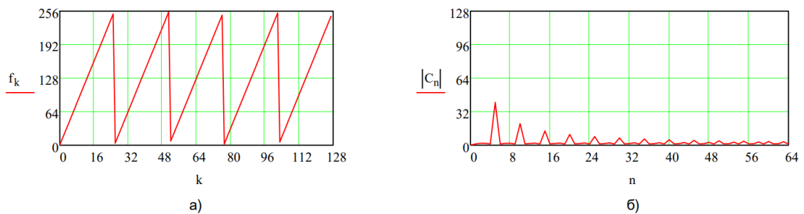
Рисунок 1 – График исходной функции (а) и её фурье-образ (б)
