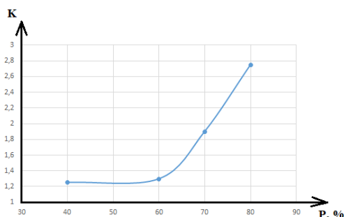
Рисунок 6 – Зависимость коэффициента K = I_{\text{ток}} / I_{\text{оптич}} от мощности
