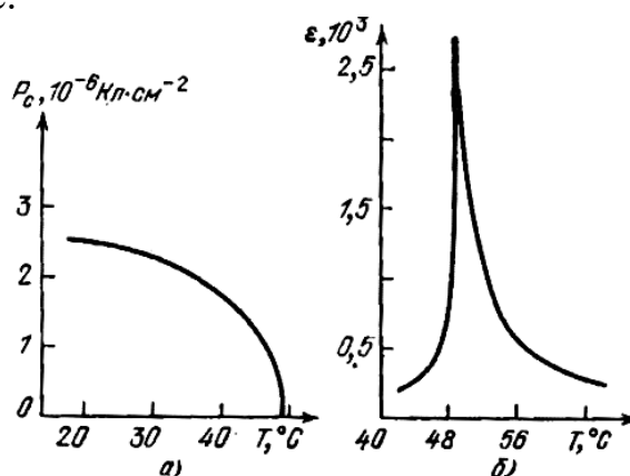
Рис. 2. Температурная зависимость спонтанной поляризации (а) и диэлектрической проницаемости (б) вдоль полярной оси 2 кристалла ТГС.
