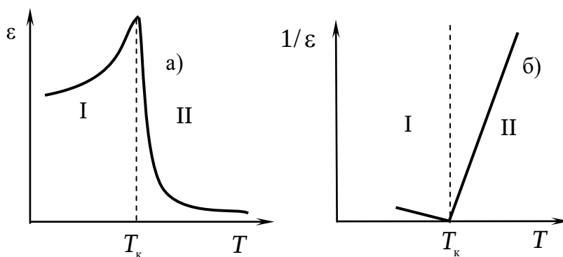
Рис. 3. I – сегнетоэлектрическая фаза ( T < T_K ); II – параэлектрическая фаза ( T > T_K ).
