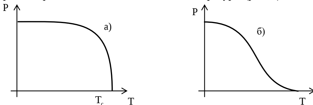
Рис. 1 а) – фазовый переход первого рода; б) – фазовый переход второго рода.
