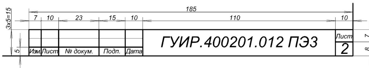
Рисунок 2.6 – Основная надпись по форме 2а
