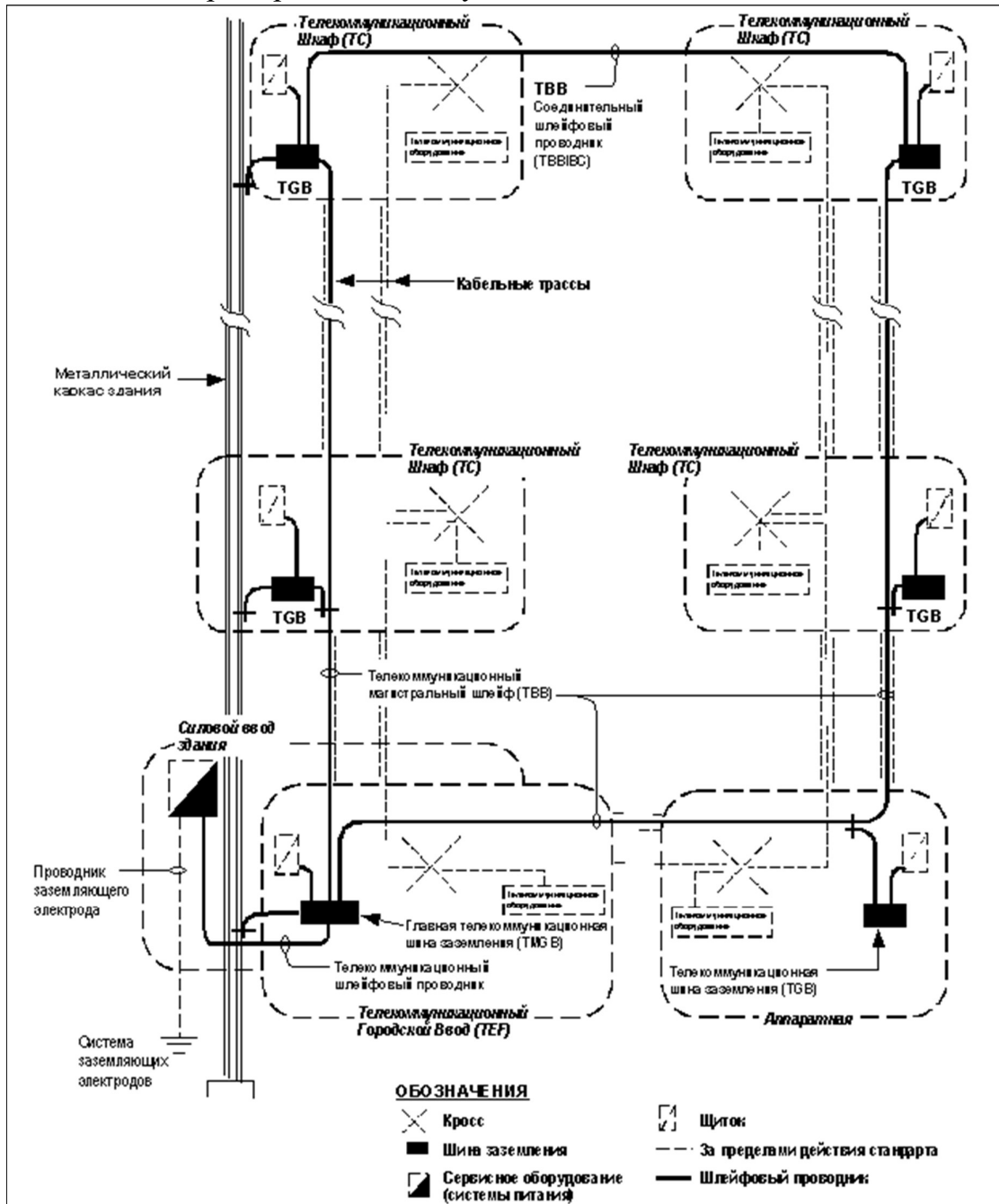
Пример схемы коммуникационного заземления
