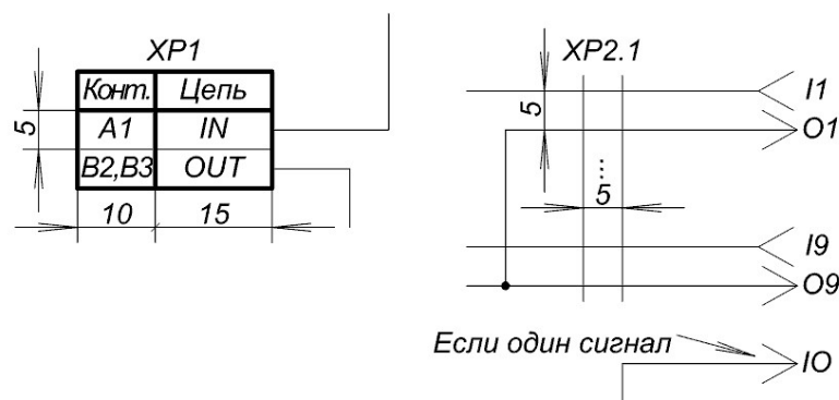
Рисунок 2.11 – Стили изображения УГО разъемов
