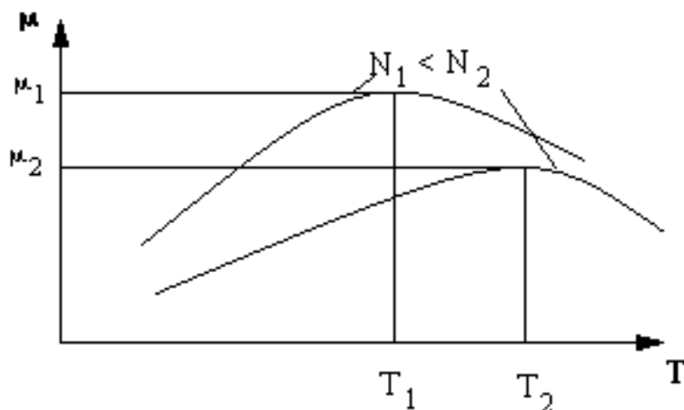
Рисунок 4.4 - Температурная зависимость подвижности носителей заряда в полупроводниках
