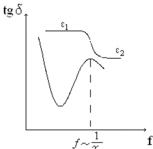
Рисунок 2.5 - Частотная зависимость \operatorname{tg} \delta
