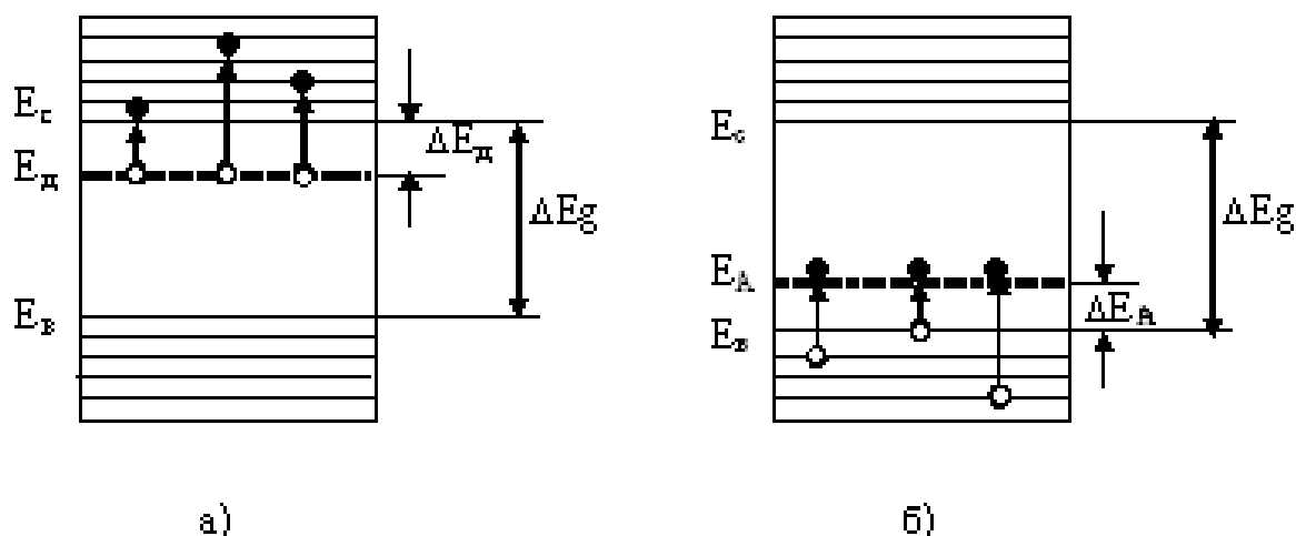
Рисунок 4.2 - Энергетические диаграммы примесных полупроводников а- донорного, б- акцепторного
