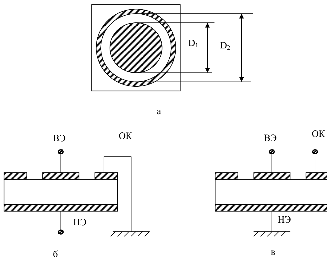
Рисунок 1.3 - Конструкция экспериментальных образцов
