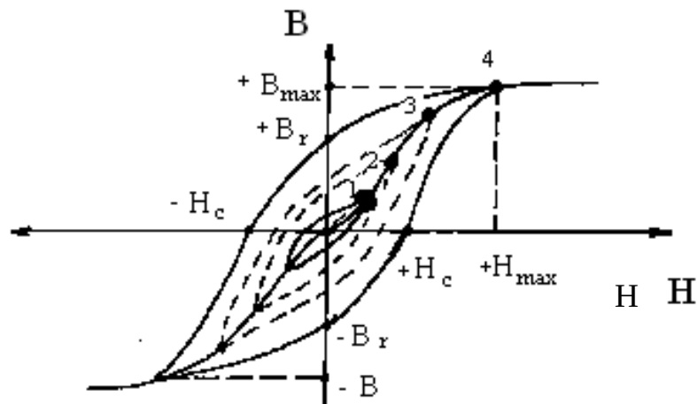
Рисунок 3.3 - Кривая перемагничивания магнетика в переменном магнитном поле
