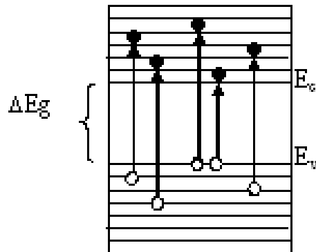
Рисунок 4.1 - Энергетическая диаграмма собственного полупроводника
