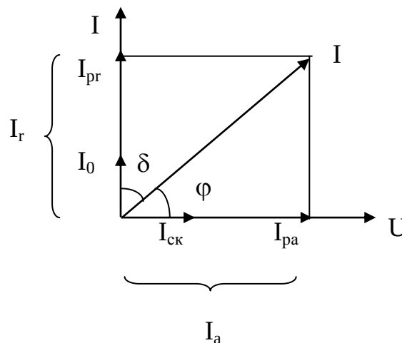
Рисунок 2.4 - Векторная диаграмма напряжения и токов в диэлектрике
