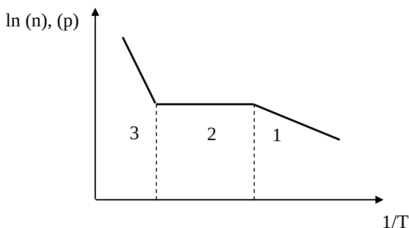
Рисунок 4.3 - Температурная зависимость концентрации носителей заряда примесного полупроводника
