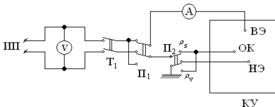
Рисунок 1.2 - Схема измерения \rho_v и \rho_s
