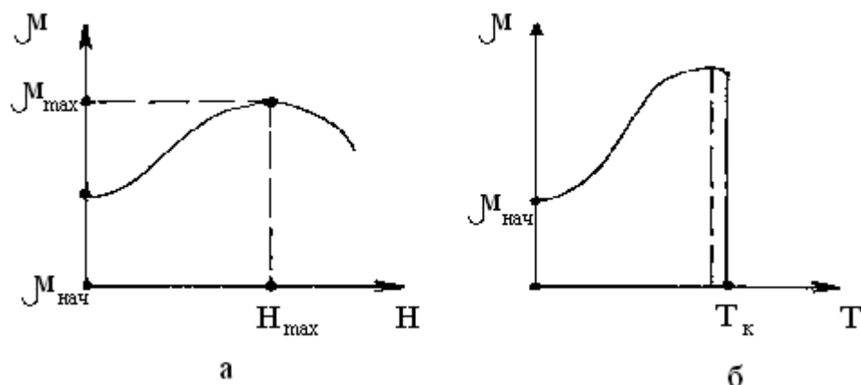
Рисунок 3.2 - Зависимость магнитной проницаемости от напряжённости внешнего поля (а) и температуры (б)
