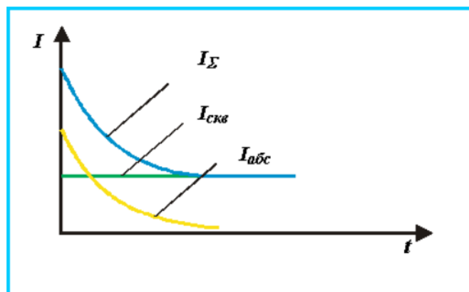
Рисунок 1.1 - Зависимость тока в диэлектрике при подключении к источнику постоянного напряжения
