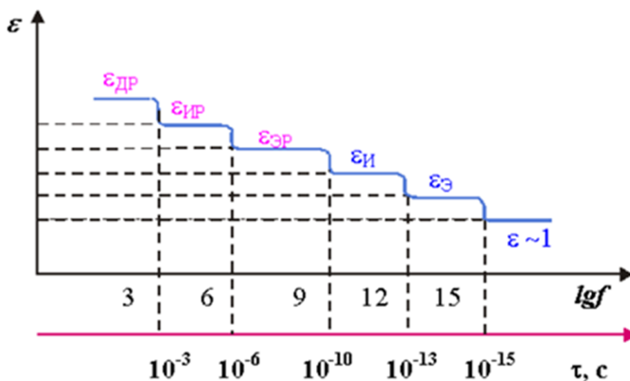
Рисунок 2.3 - Дисперсия диэлектрической проницаемости
