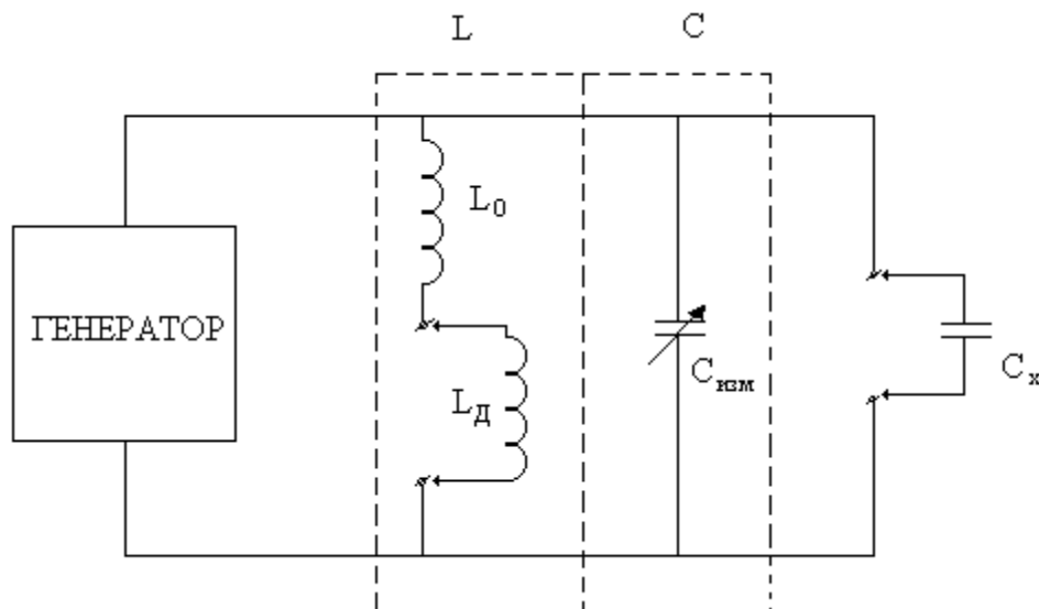
Рисунок 2.6 - Упрощенная схема измерителя добротности Е4-7
