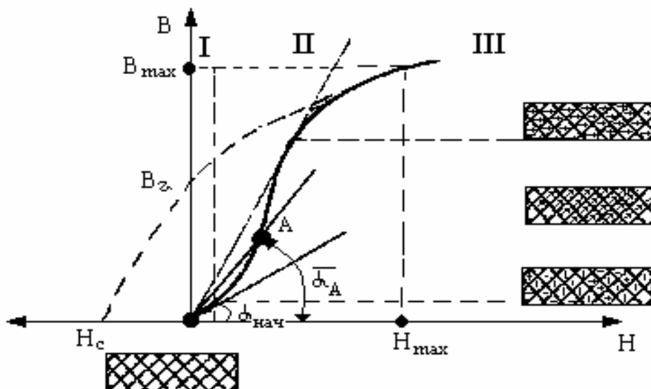
Рисунок 3.1 - Кривая намагничивания магнетика и схематическое положение магнитных моментов на разных стадиях намагничивания
