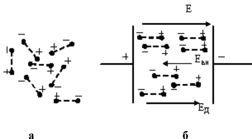
Рисунок 2.2 - Расположение зарядов в диэлектрике: а - в отсутствие внешнего поля; б - при приложении внешнего поля
