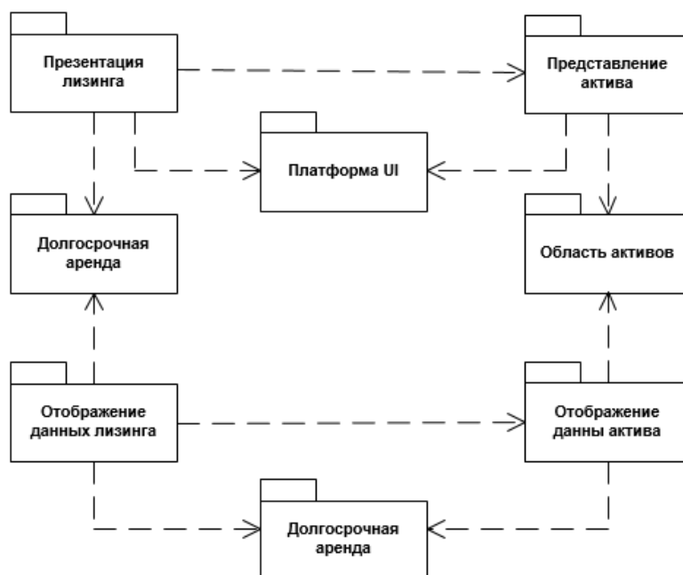
Рисунок 3.8 – Диаграмма пакетов
