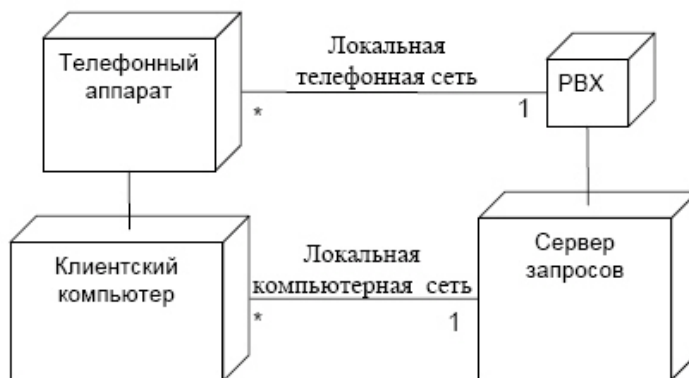
Рисунок 3.7 – Диаграмма развертывания
