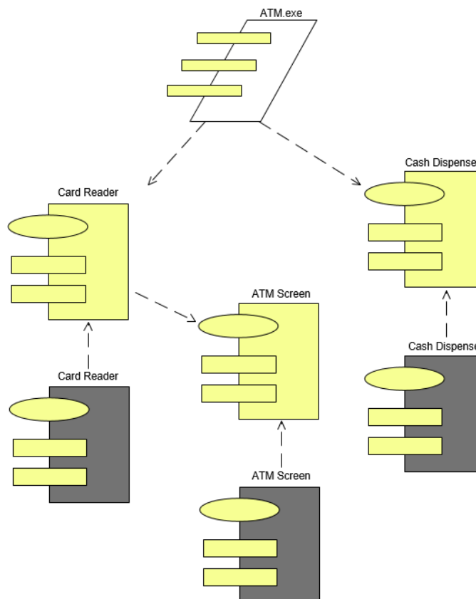
Рисунок 3.5 – Диаграмма компонентов
