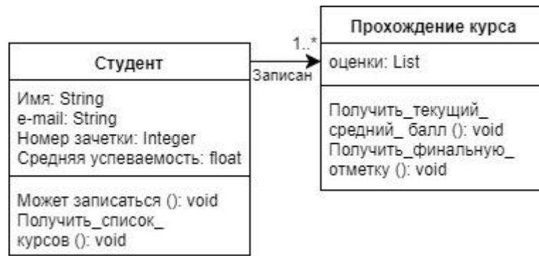
Рисунок 3.4 – Диаграмма классов
