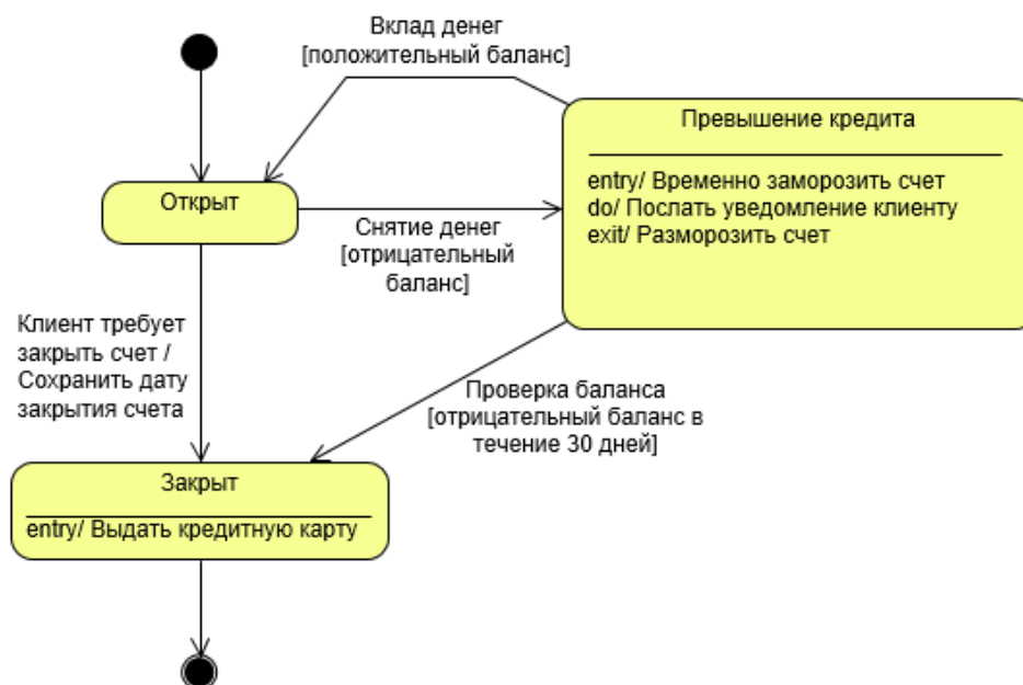
Рисунок 3.9 – Диаграммы активности
