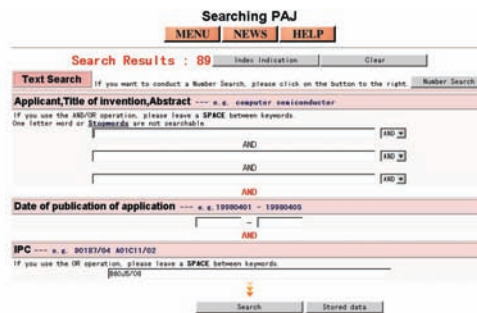
Рис. 45. Результаты поиска
