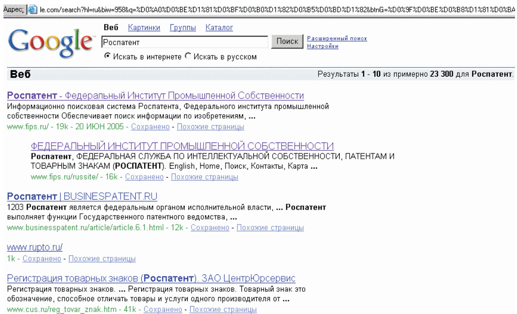
Рис. 2. Результаты поиска
