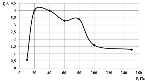
Рис. 1 – График зависимости величины тока разряда от величины давления плазмообразующей среды при напряжении U = 600 В, скважность импульсов Q = 10 , частоте следования импульсов f = 5 кГц
