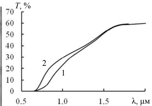
Рис. 2 – Спектры пропускания стекол с наночастицами: 1 – \text{CuInTe}_2 ; 2 – \text{CuGaTe}_2
