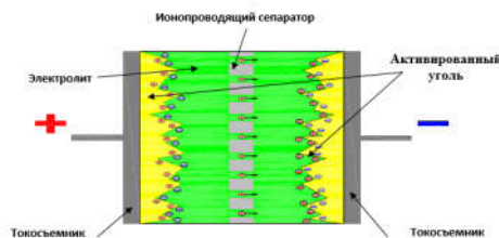
Рис. 1 - Принципиальная схема суперконденсатора
