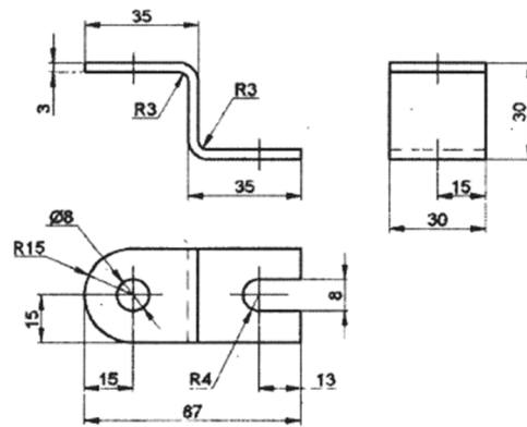
Рисунок 1. – Эскиз кронштейна
