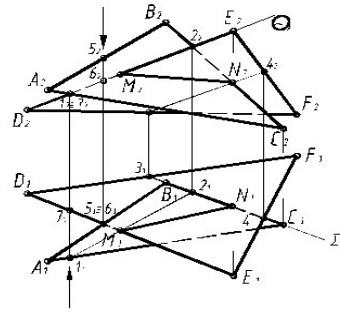
Рис. 2 – Пересечение плоскостей
