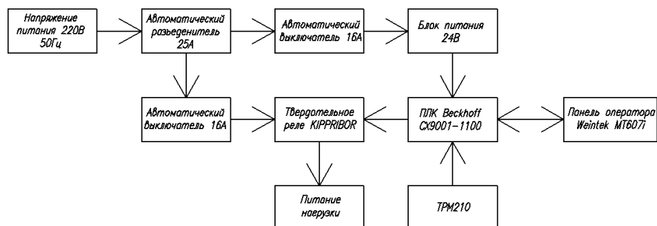
Рис. 1. Структурная схема управления ВЧ инвертором
