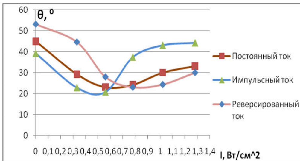
Рис. 3. Зависимости угла смачивания от интенсивности УЗК
