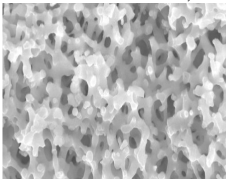
Рисунок 4 – Углеродная нанопена
