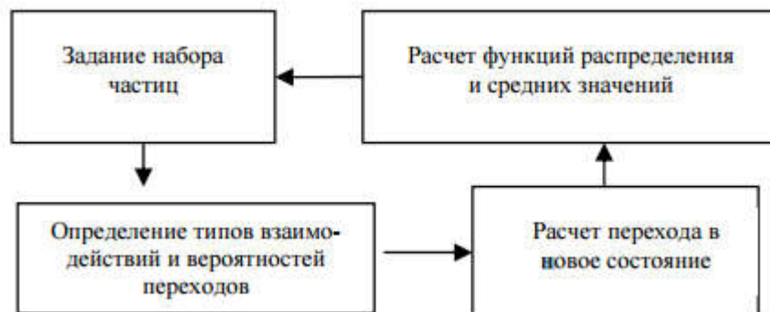
Рис.1 Общая схема метода Монте-Карло.
