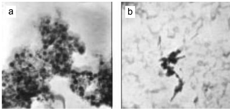
Рис. 1 – Микрофотографии частиц \text{CuInTe}_2 , сформированных в стекле без термообработки (а) и после термообработки (6 ч) при температуре 550 °С (б). Увеличение: 40000
