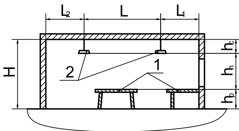
Рис. 4. Разрез помещения:
