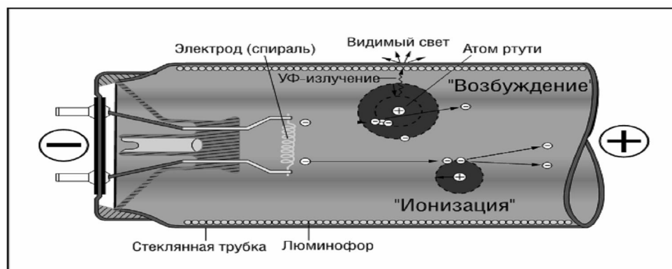
Рисунок 2. Принцип генерации света в люминесцентных лампах на примере лампы с термокатодом
