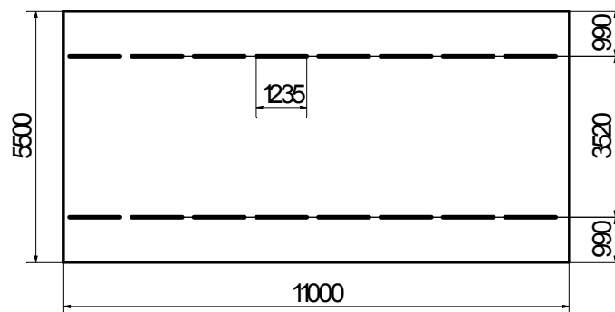
Рис. 5. Размещение светильников на плане помещения.
