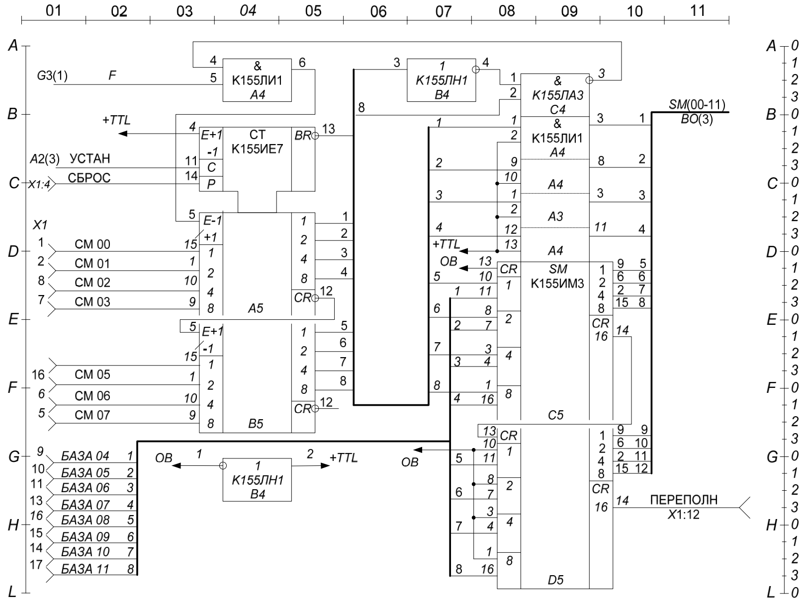
Рисунок 3.45 – Фрагмент схемы электрической принципиальной при делении поля листа на зоны
