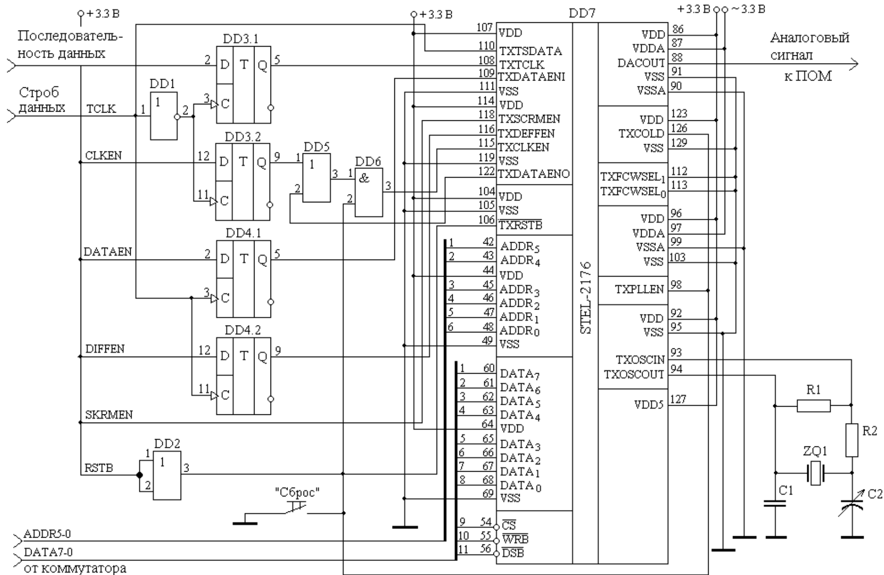
Рисунок 3.44 – Фрагмент принципиальной электрической схемы цифрового устройства
