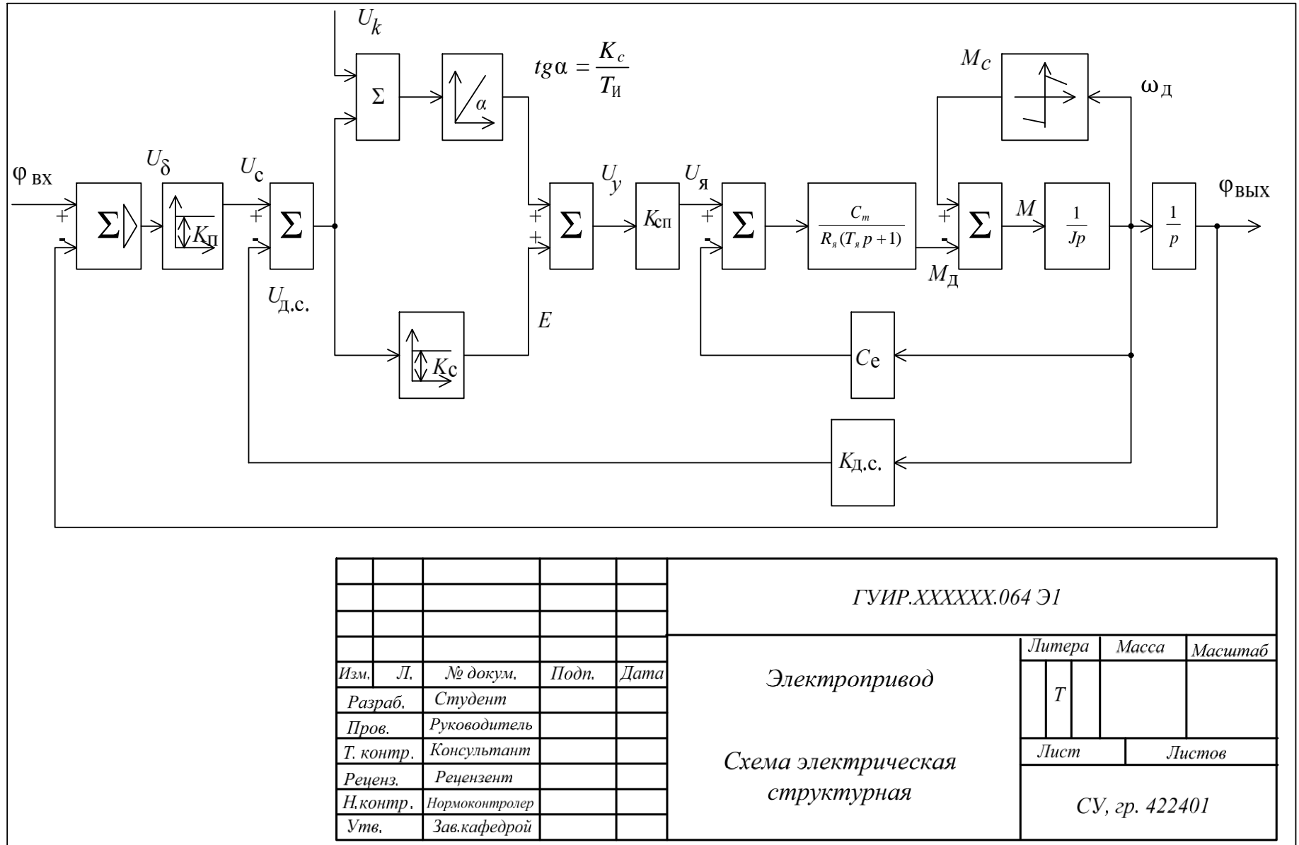
Рисунок 3.19 – Пример оформления схемы электрической структурной электропривода на чертеже
