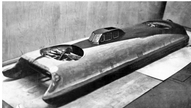
Макет катера на воздушной подушке Л-1
